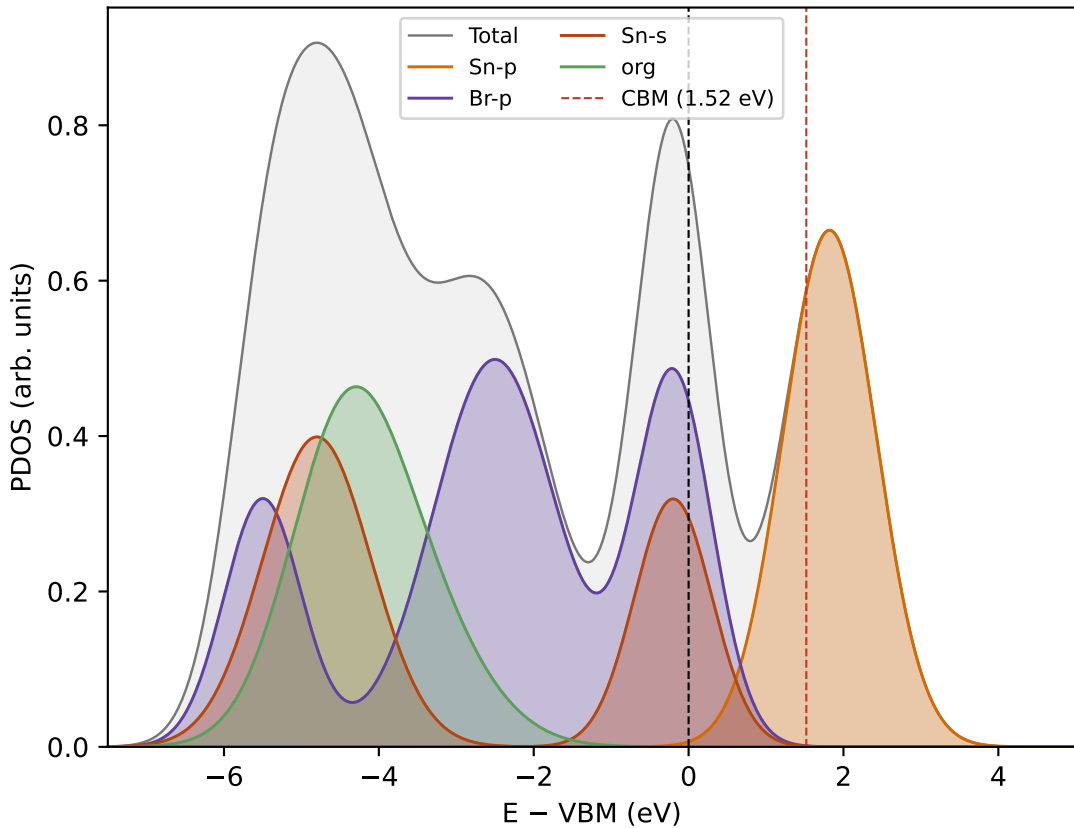
FASnBr3 — PDOS Al (campo cristalino)
