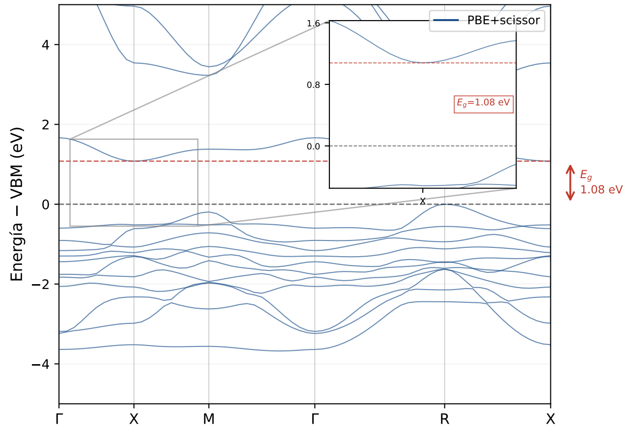
Estructura de bandas — FAPbBr 3 (PBE+scissor)
