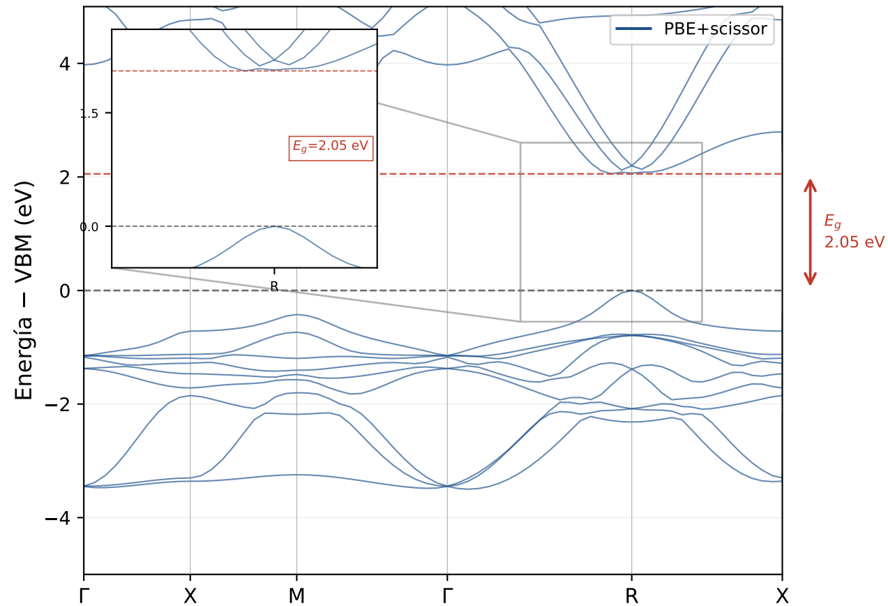
Estructura de bandas — MAPbI 3 (PBE+scissor)
