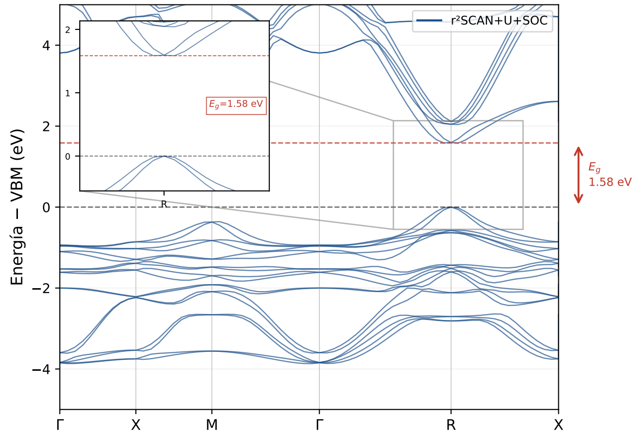
Estructura de bandas — MASnI 3 (r 2 SCAN+U+SOC)
