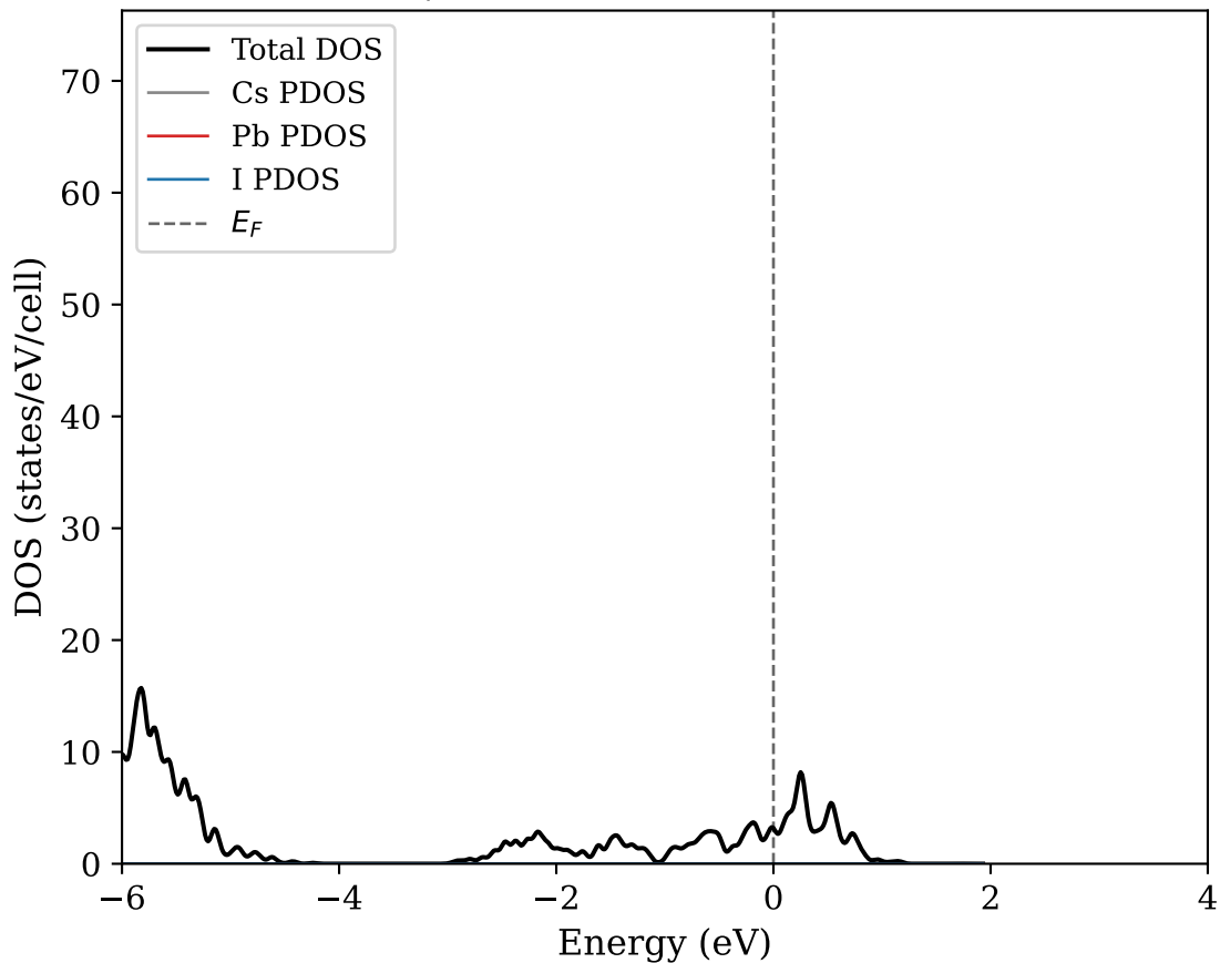
\alpha -CsPbI 3 | Total DOS + PDOS (PBE, 12×12×12)
