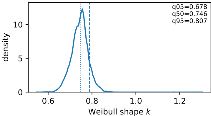
rf-abc-rnpe: posterior of k
