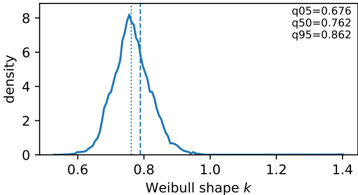
prnpe: posterior of k
