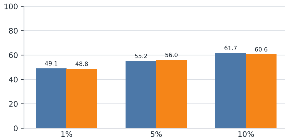
SQuAD v2 F1 Score
