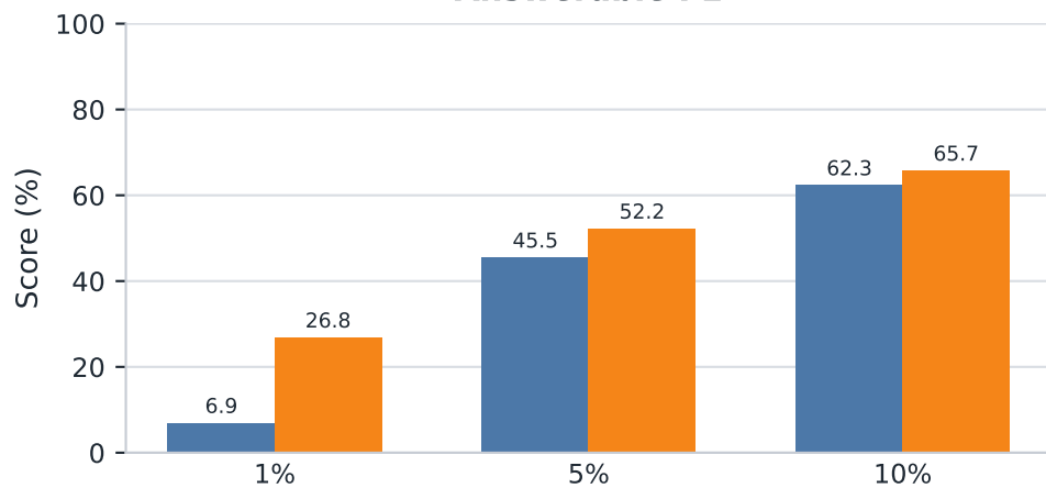
SQuAD v2 Answerable F1
