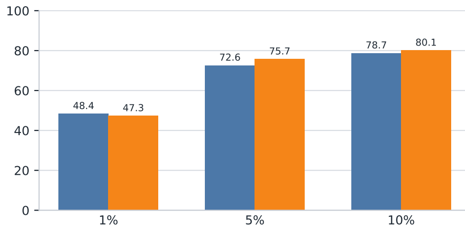
SQuAD 1.1 F1 Score
