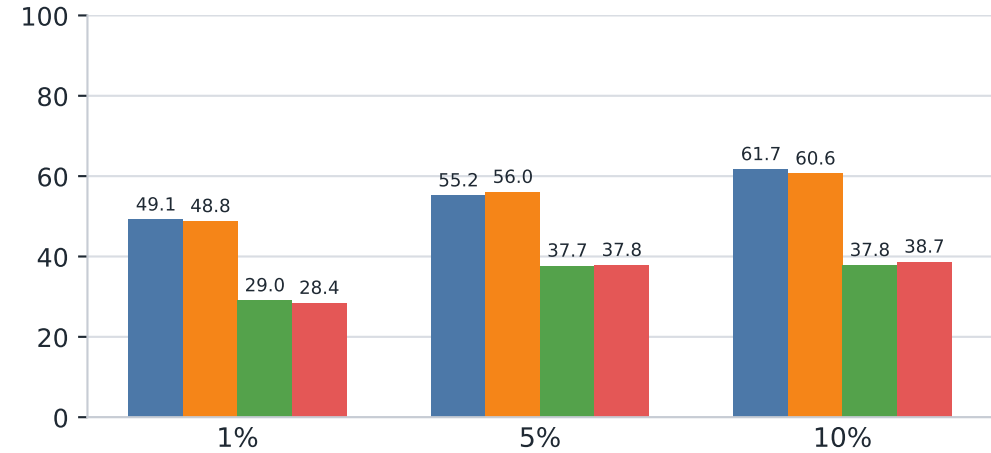
SQuAD v2 F1 Score
