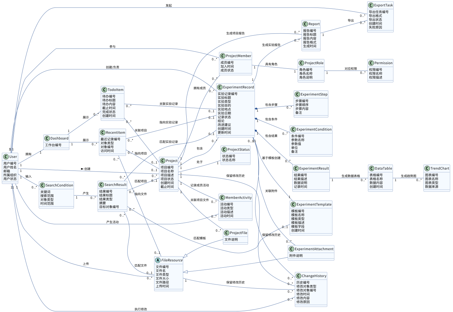
BioNote 生物实验记录助手 - 概念类图
