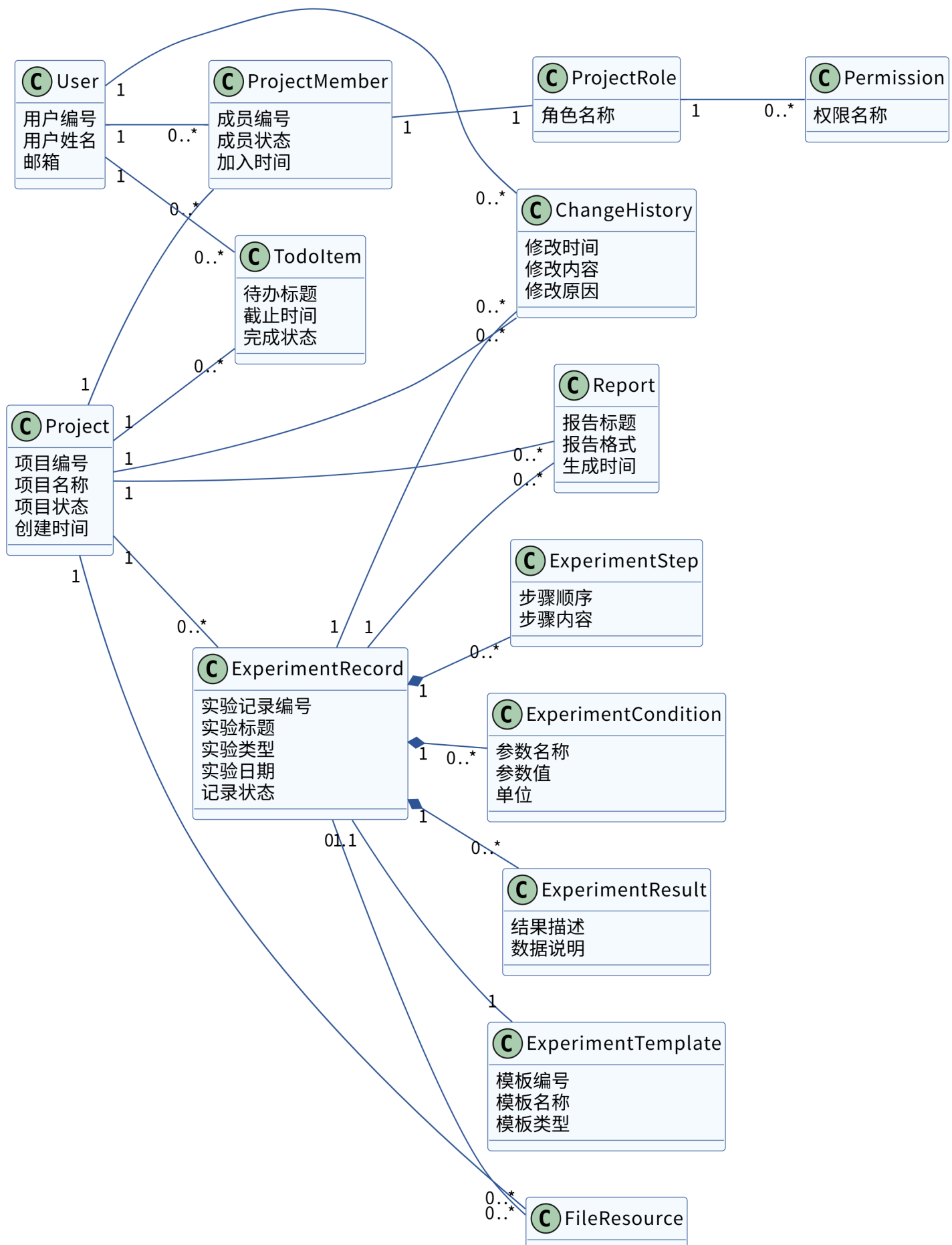
BioNote 生物实验记录助手 - 简化概念类图
