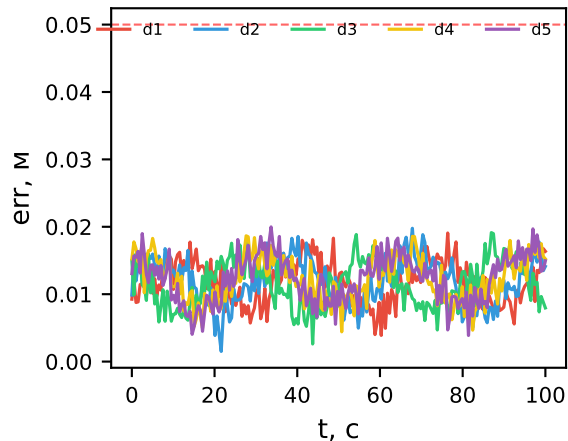
SLAM error per drone (m)
