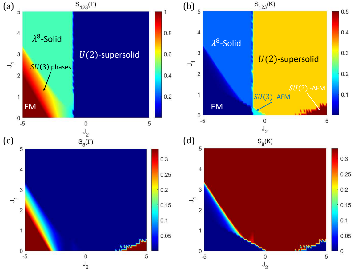
图 5.5 U(2) \times T 模型在全部参数空间中 \lambda^{123} 与 \lambda^8 的结构因子在 \Gamma, K 点的分布。(a-d) 分别是 S_{\lambda^{123}}(\Gamma), S_{\lambda^{123}}(K), S_{\lambda^8}(\Gamma), S_{\lambda^8}(K) 在各个参数点的分布。
