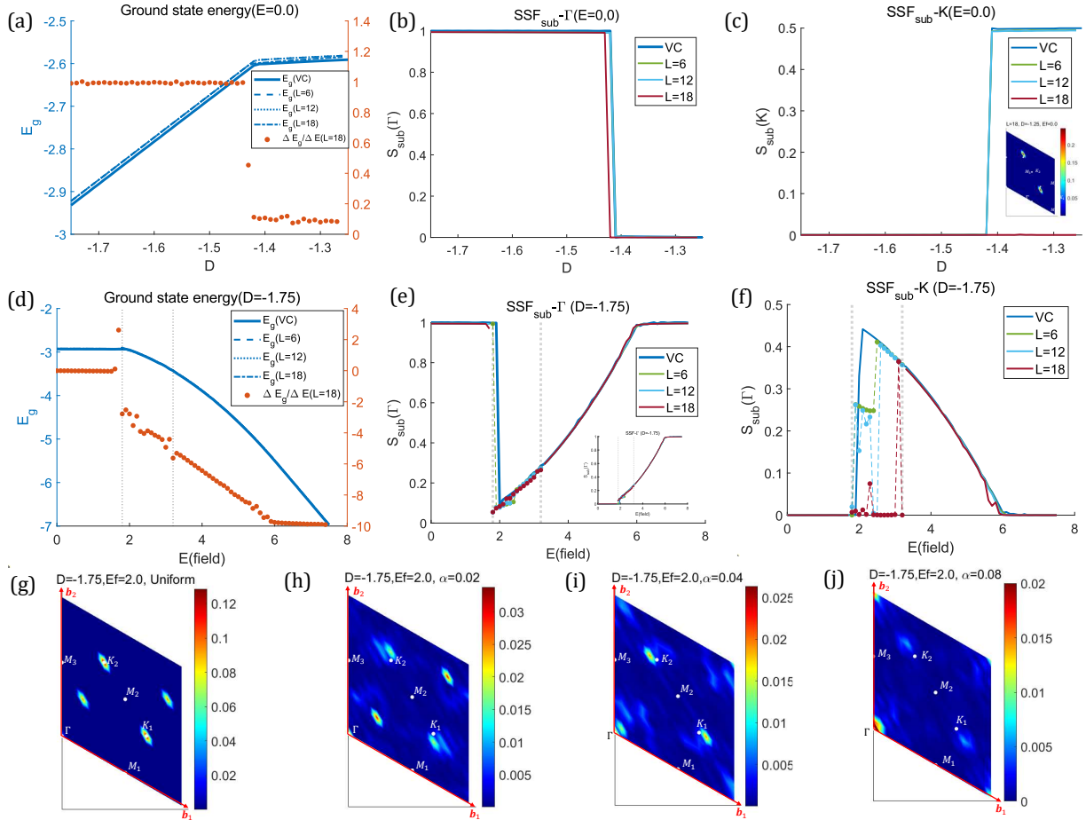
图 4.2 \alpha - \text{RuCl}_3 唯象电偶极模型(4.6)的蒙特卡洛模拟的若干结果。(a-c) 零场下基态随各向异性势 D 的变化, 蒙特卡洛模拟晶格尺寸为 L = 6, 12, 18 , 温度设置为 T/k_B = 0.01 : (a) 不同各向异性势 D 下格点平均能量的系综平均变化曲线, 其中实线为用于对比的变分计算能量曲线(VC), 红色散点为 L = 18 尺寸下格点平均能量的一阶差分; (b) 不同各向异性势 D 下 \Gamma 点电偶极子格结构因子 S^{(\text{sub})}(\Gamma) 变化曲线, 其中深蓝色实线为用于对比的变分计算结果; (c) 电偶极子格结构因子的 K 点数值 S^{(\text{sub})}(K) 变化曲线(小图: L = 18, D = -1.25 时的子格结构因子 S^{(\text{sub})}(q) 在等效第一布里渊区的完整分布)。(d-f) 固定各向异性势 D = -1.75 下, 基态随匀强外场 E 的变化, 蒙特卡洛模拟尺寸与温度设置与(a-c)一致, 在 -1.8 \leq E \leq 3.2 电场区间的预测数据用散点标注: (d) 不同电场强度 E 下格点平均能量的系综平均变化曲线; (e) \Gamma 点的电偶极子格结构因子 S^{(\text{sub})}(\Gamma) 变化曲线(小图: \Gamma 点的晶格结构因子在 \Gamma 点取值 S^{(\text{sub})}(\Gamma) 的变化曲线); (f) K 点的电偶极子格结构因子变化曲线 S^{(\text{sub})}(K) 。(g-j) D = -1.75, E_0 = 2 参数点不同电场分布展宽下的子格结构因子 S^{(\text{sub})}(q) 在等效第一布里渊区的分布, 倒格矢方向已标注图中, 分别为 \alpha = 0, 0.02, 0.04, 0.08 , (j) 图的结构因子数值在 0.02 做了截断, \Gamma 点峰值实际可达 0.2。
