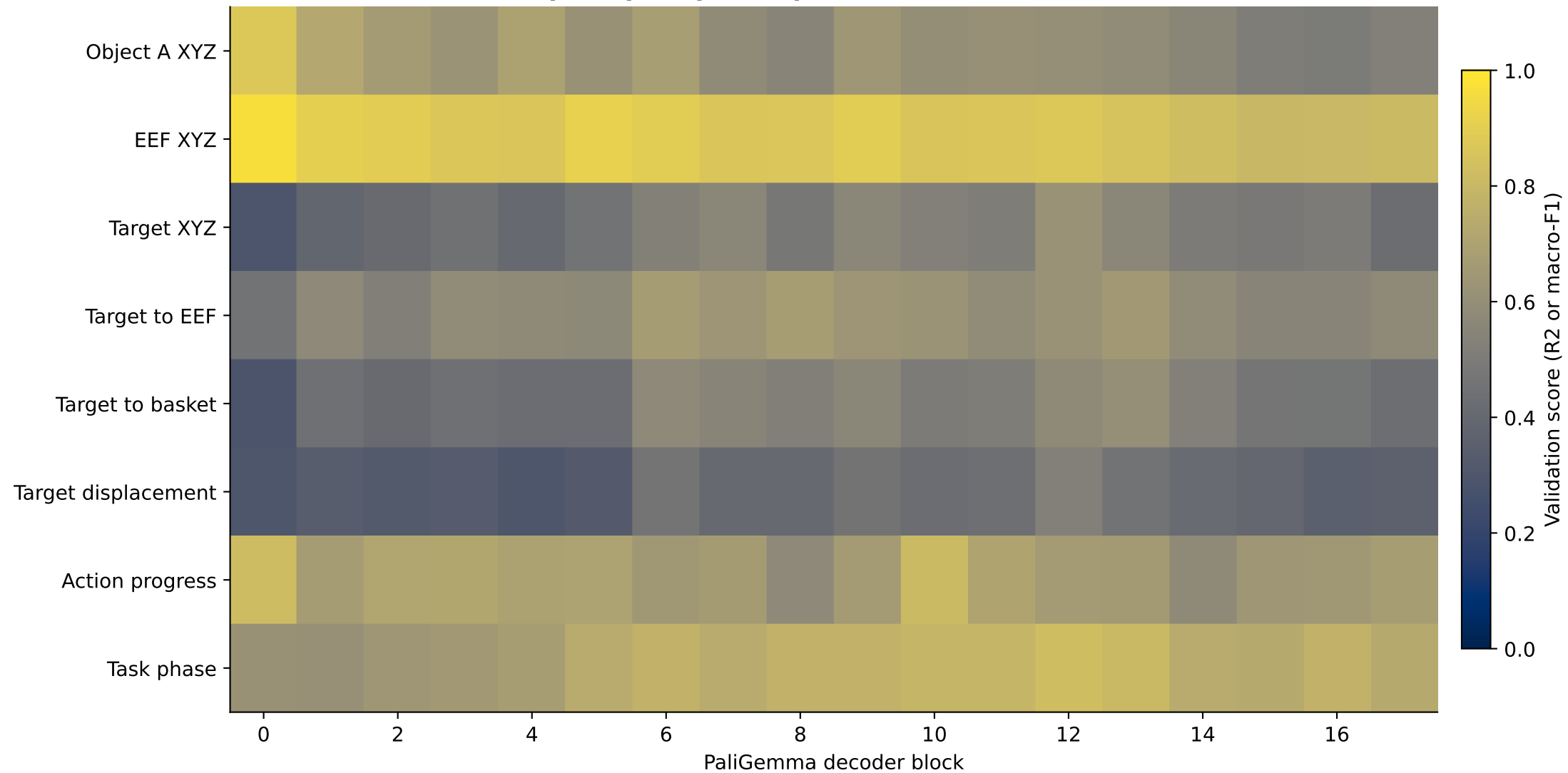
pi0.5 prompt-end paired world-state atlas
