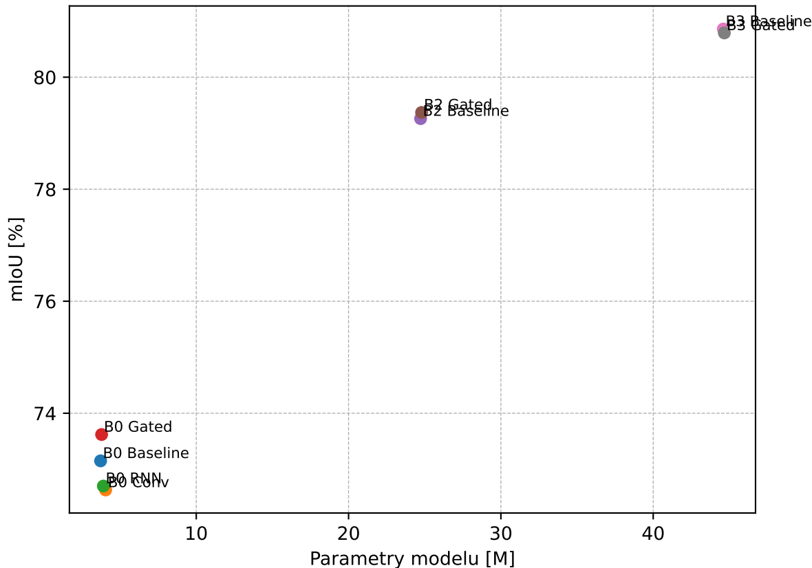
mIoU vs liczba parametrów (160k)
