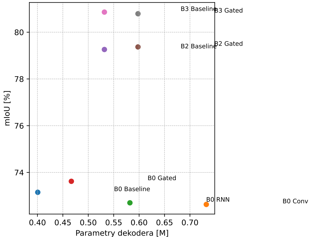
mIoU vs liczba parametrów dekodera (160k)
