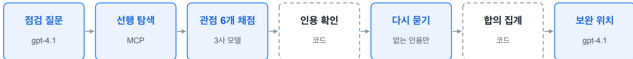
LangGraph 상태 그래프
