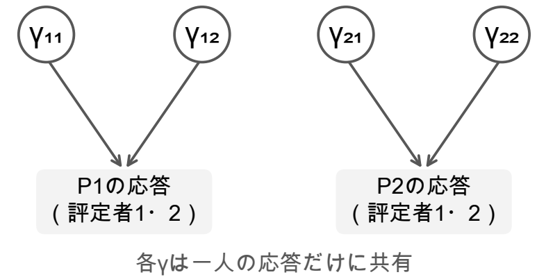
B 人×評定者の局所効果 (構造図)
