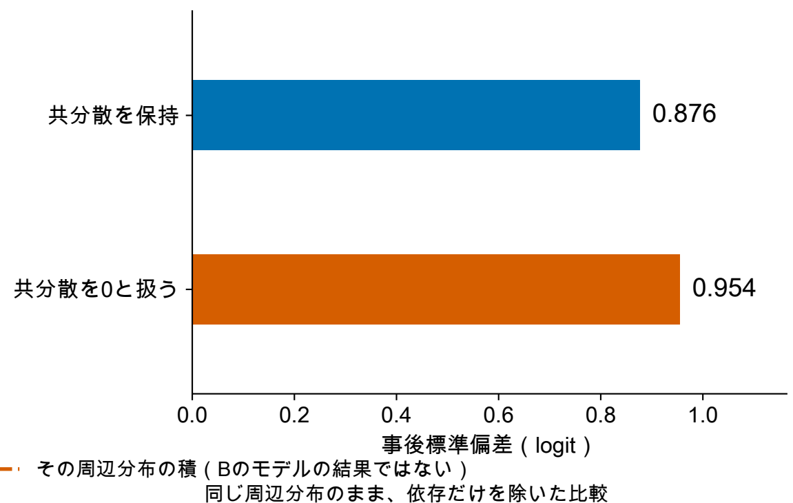
D 能力差 \theta_1 - \theta_2 の標準偏差
