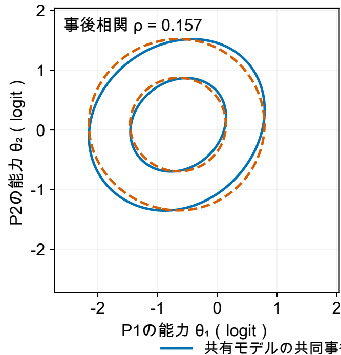
C 能力の共同事後分布
