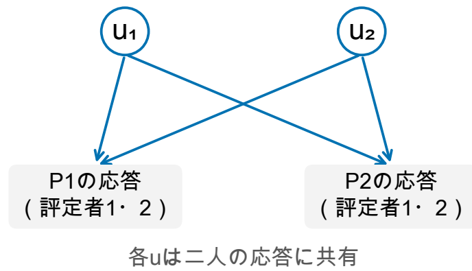
A 共有評定者効果 (系列R)
