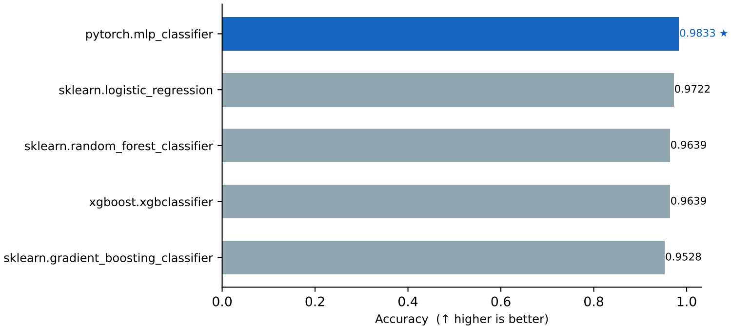
tabular.digits — Accuracy
