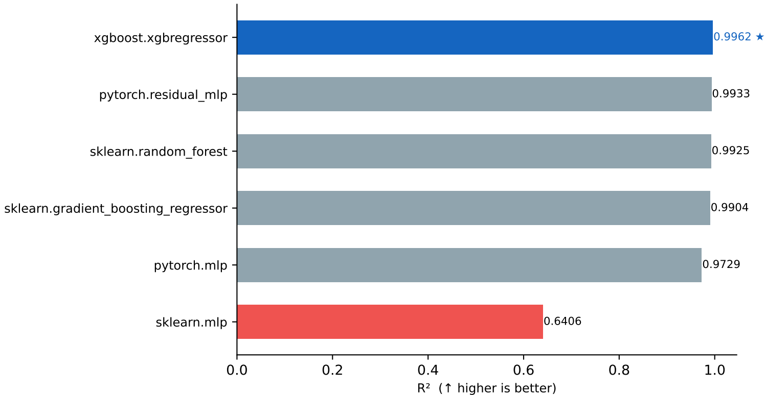
tabular.energy_efficiency — R 2
