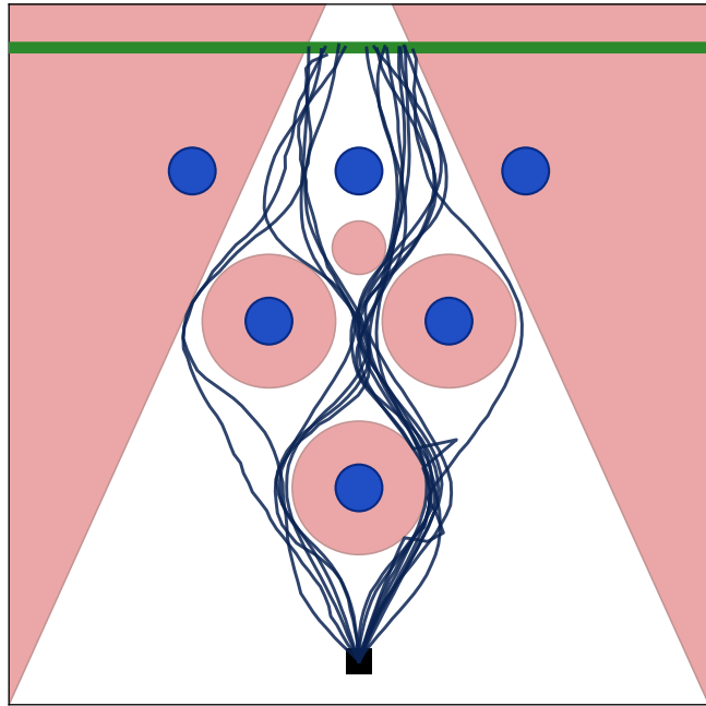
BayesFP (Ours)
