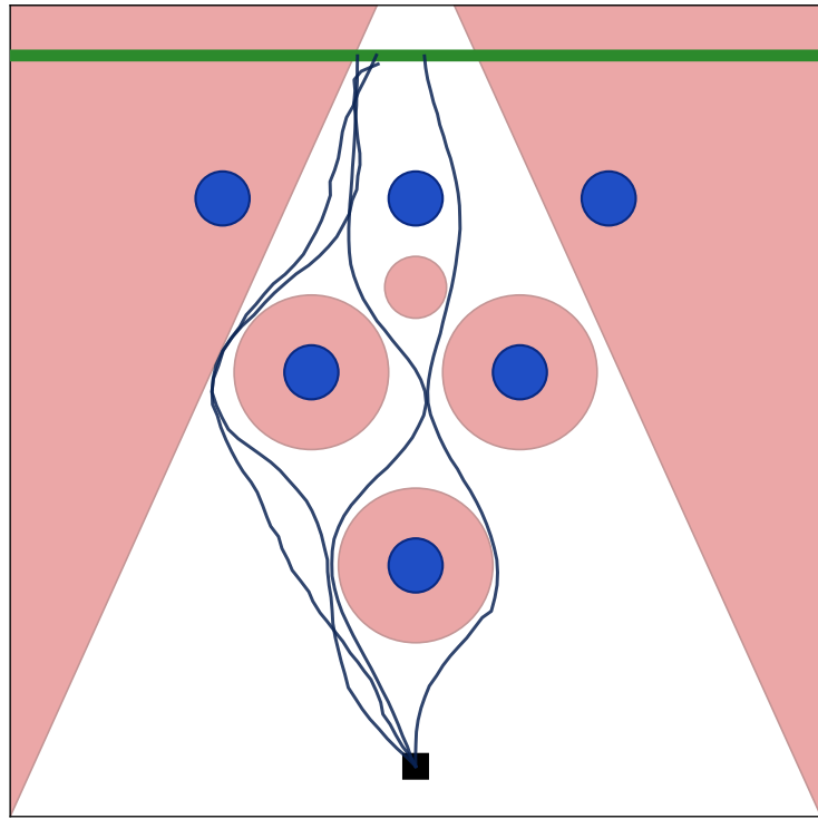
FKC (Ours)
