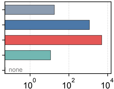
CRIU cold
