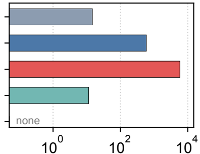
CRIU warm
