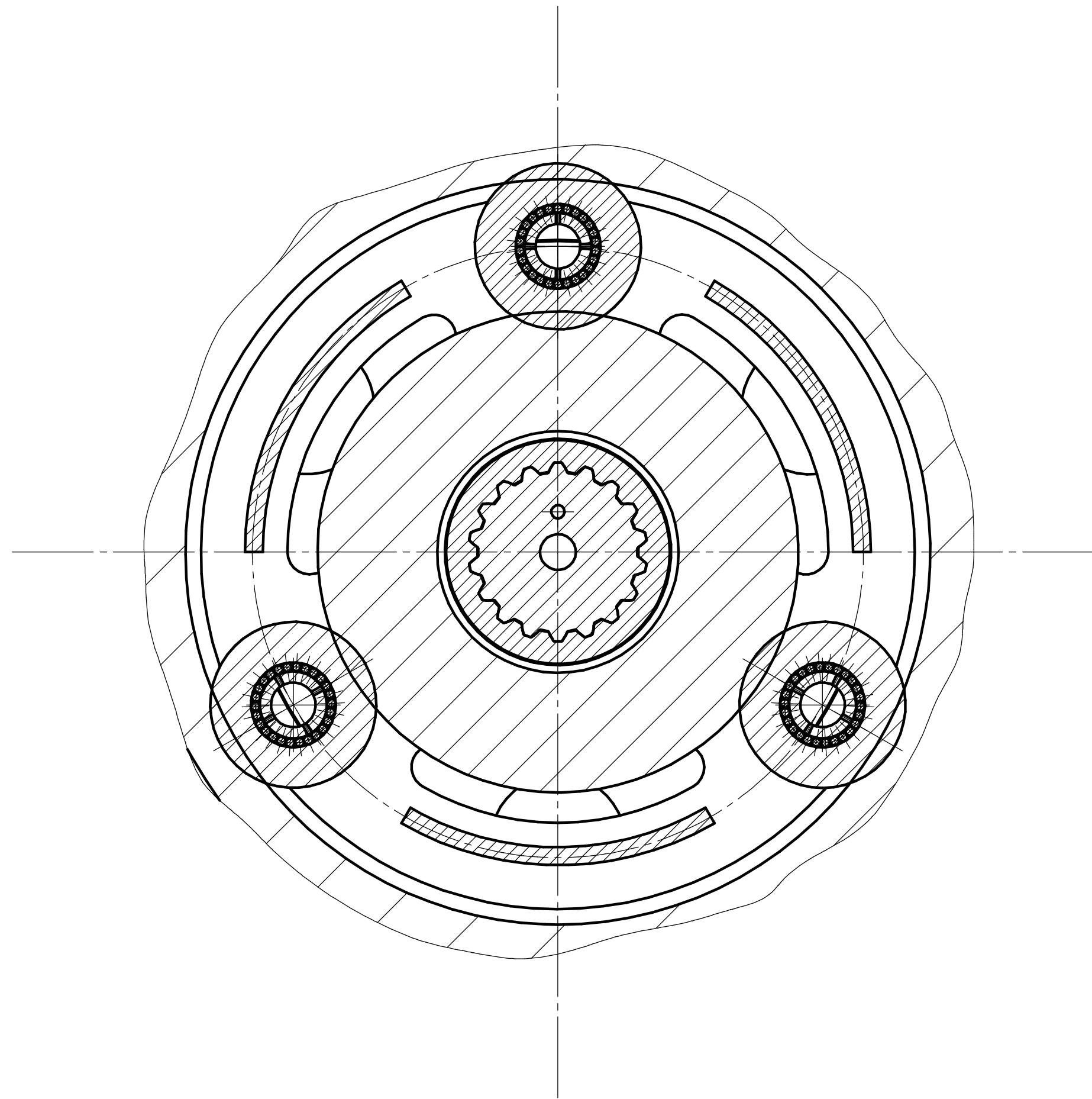
Г-Г(1:1)(2)
