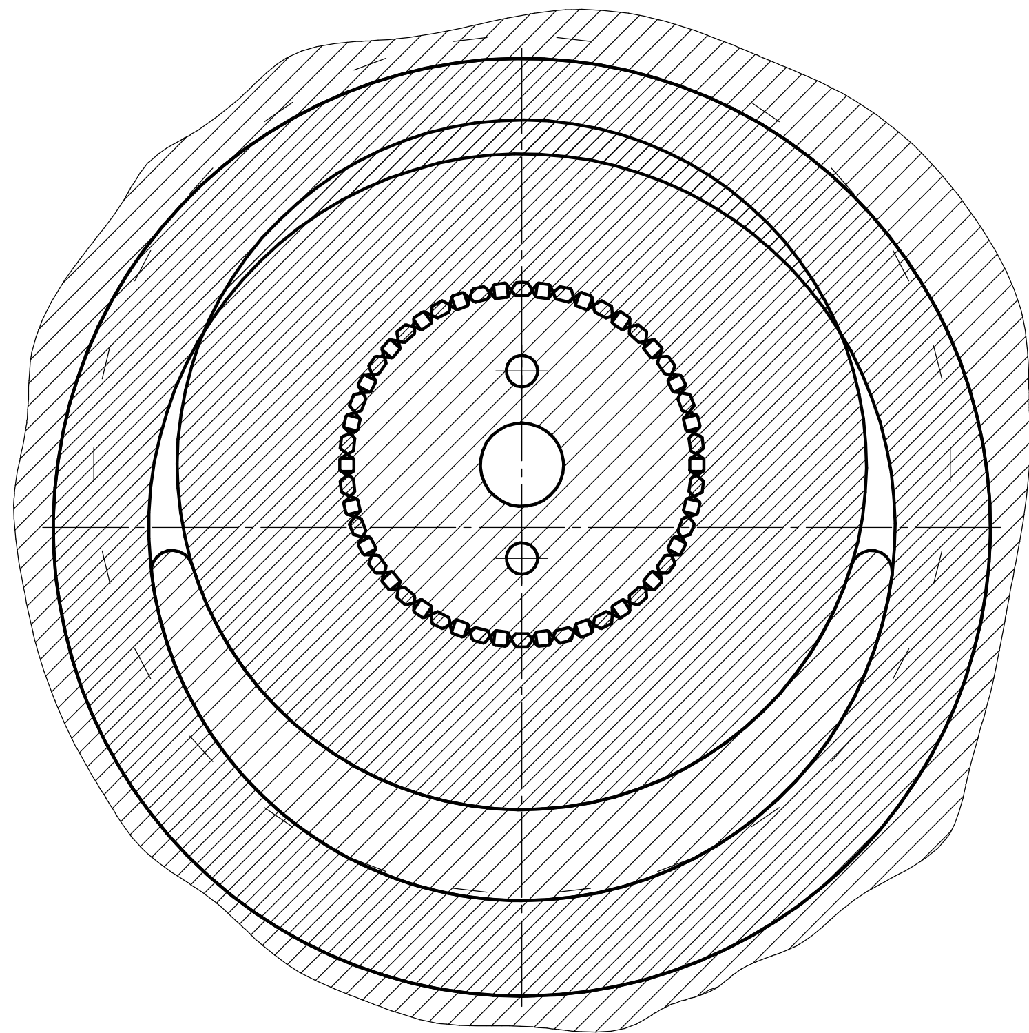
Е-Е(1:1)(2)
