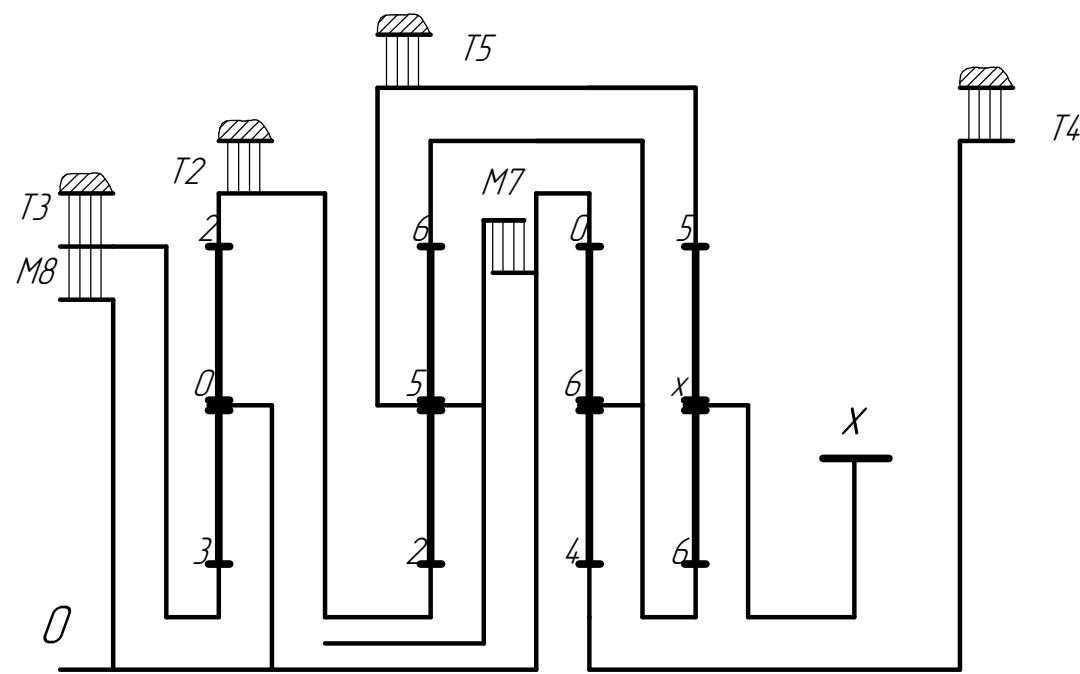
Кинематическая схема ПКП
