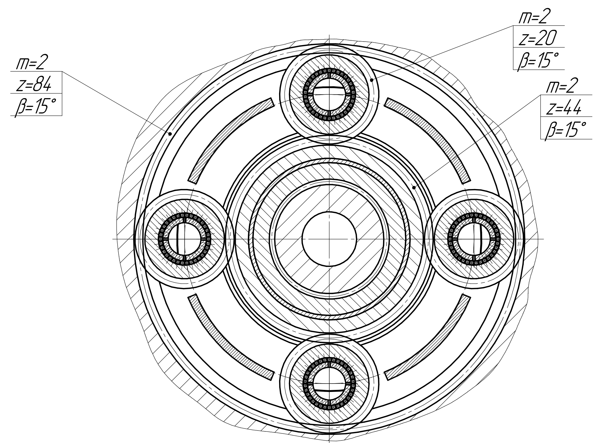
Ж-Ж(1:1)/(2)
