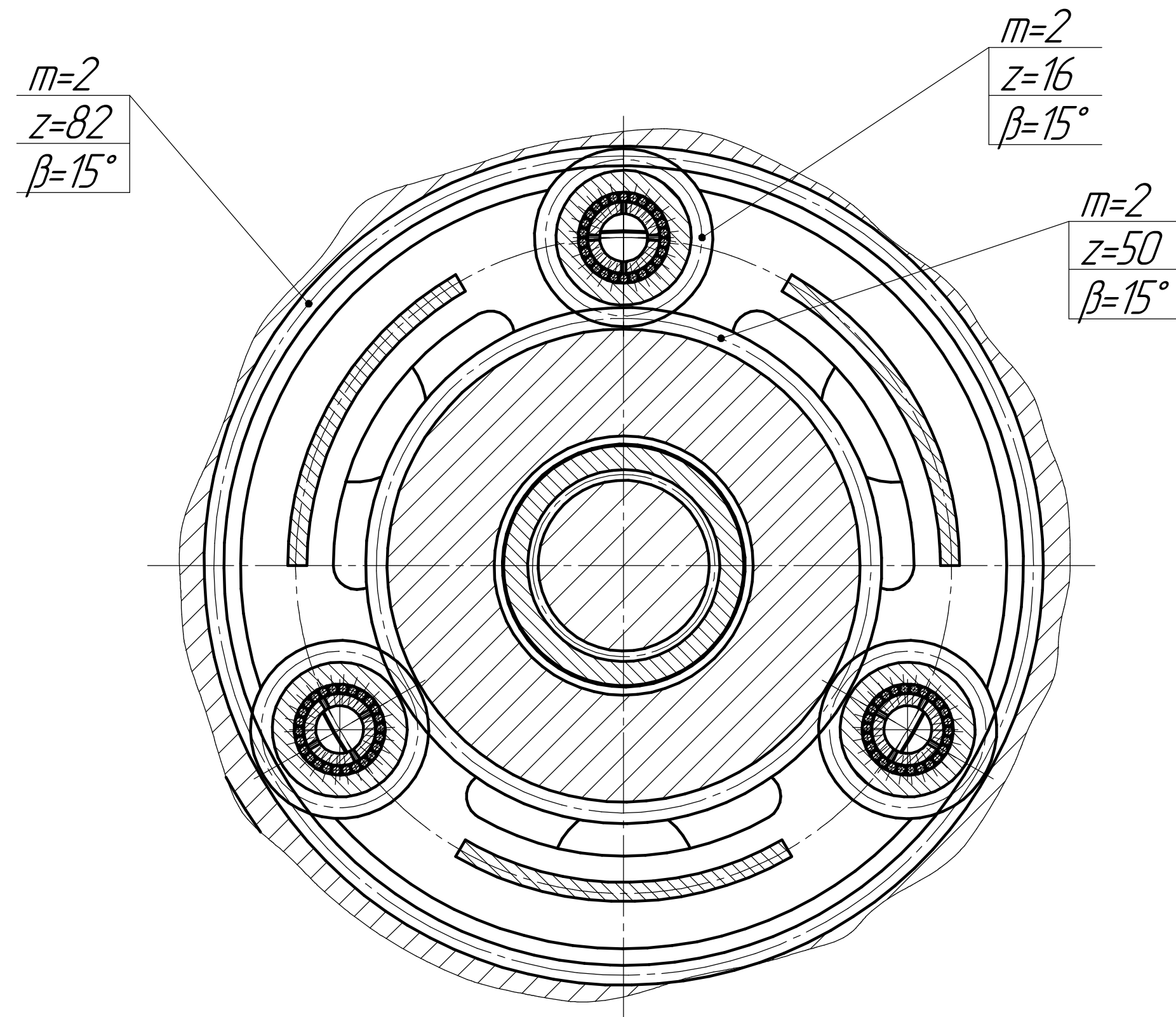
Г-Г(1:1)/(2)
