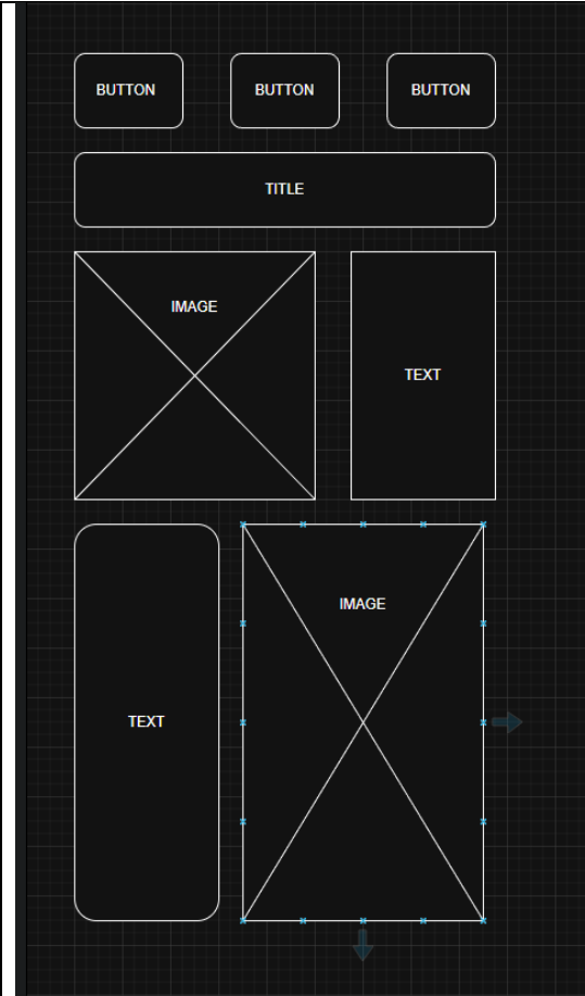
uiscelRE.html mobile
