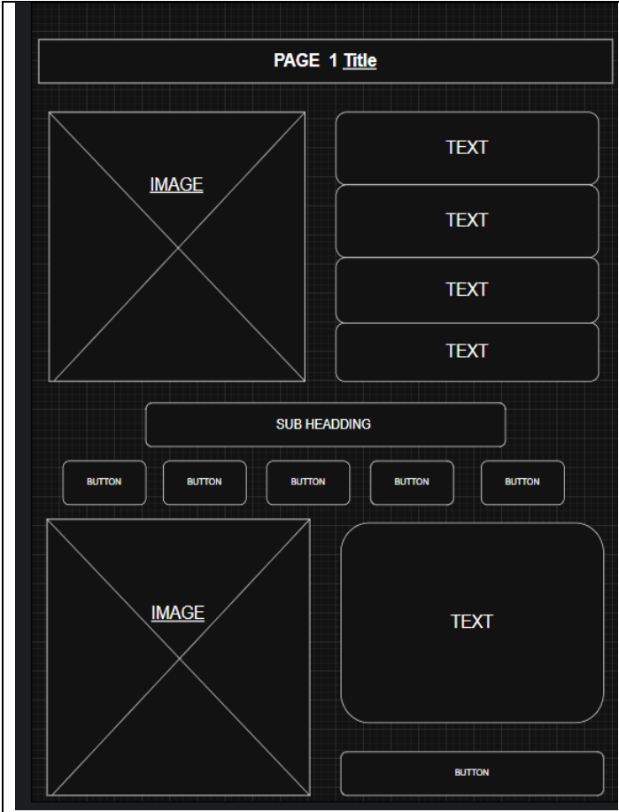
uiscelRE.html desktop
