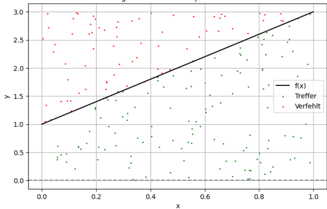
Numerische Integration mittels Monte-Carlo Ergebnis bei n=200 | \approx 1.92000
