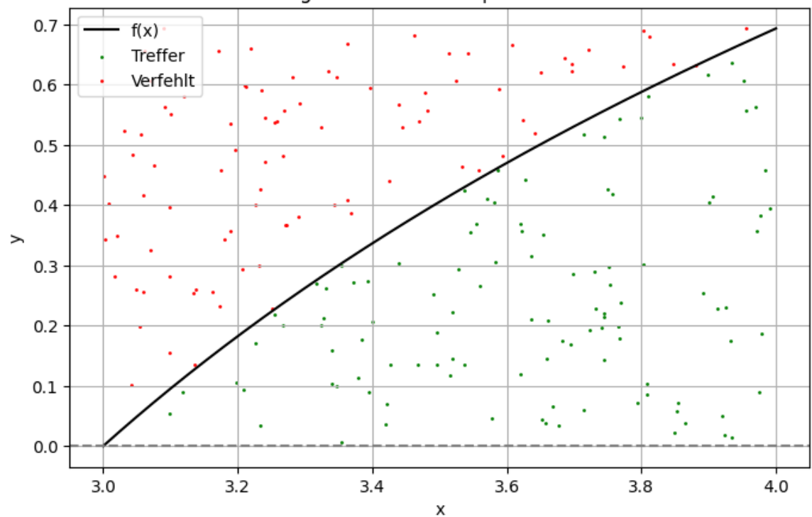
Numerische Integration mittels Monte-Carlo Ergebnis bei n=200 | \approx 0.37777
