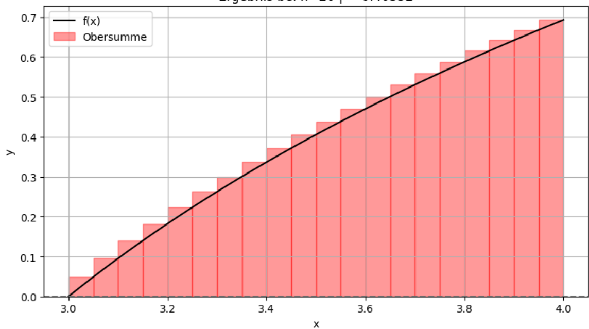
Numerische Integration mittels Obersumme Ergebnis bei n=20 | \approx 0.40352
