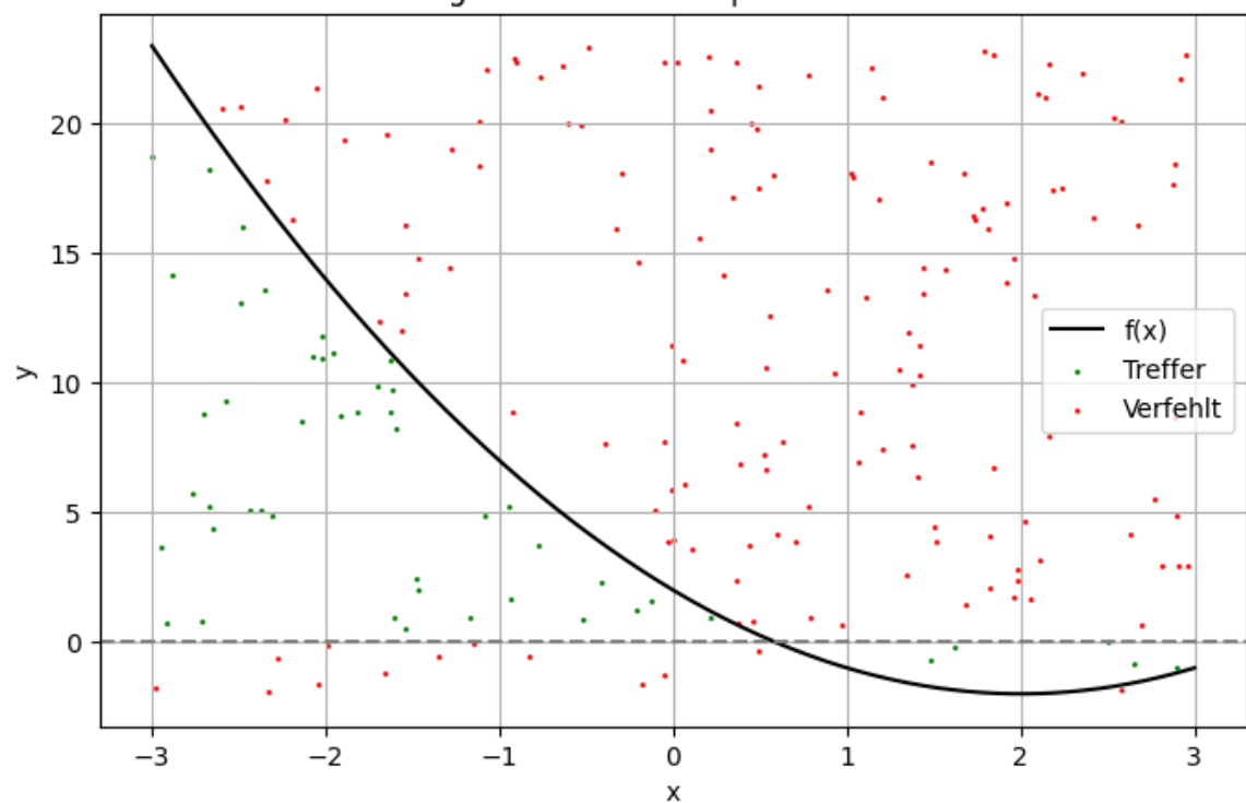
Numerische Integration mittels Monte-Carlo Ergebnis bei n=200 | \approx 28.49999
