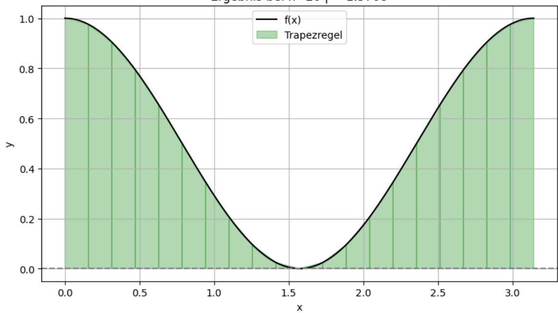
Numerische Integration mittels Trapezregel Ergebnis bei n=20 | \approx 1.5708
