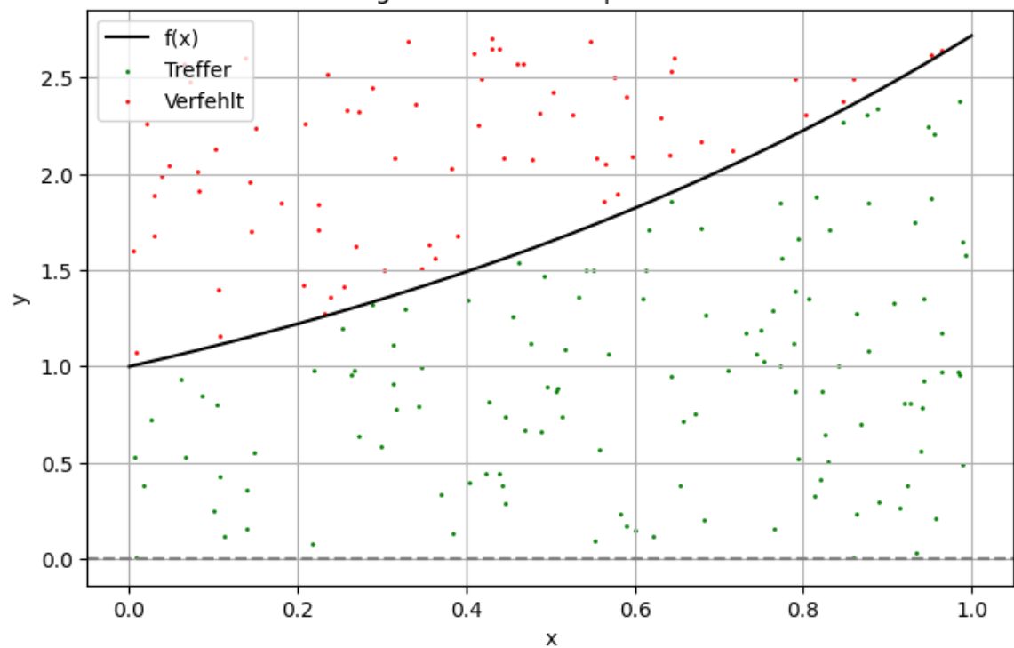
Numerische Integration mittels Monte-Carlo Ergebnis bei n=200 | \approx 1.72611
