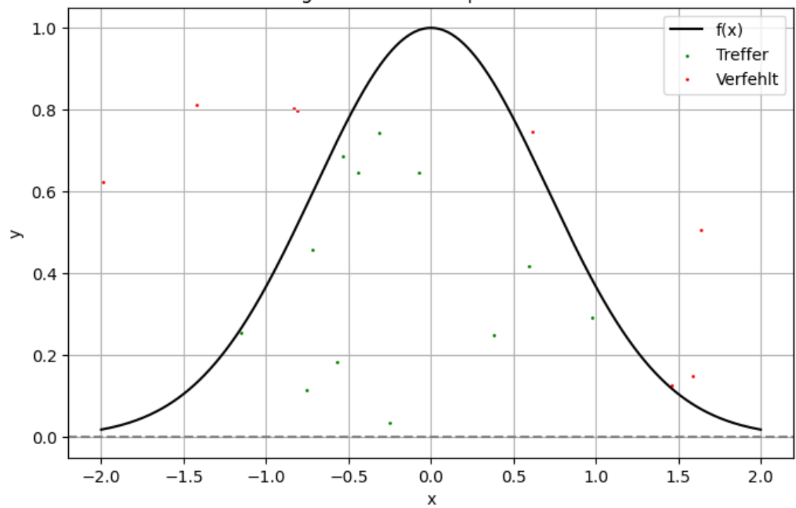
Numerische Integration mittels Monte-Carlo Ergebnis bei n=20 | \approx 2.39999
