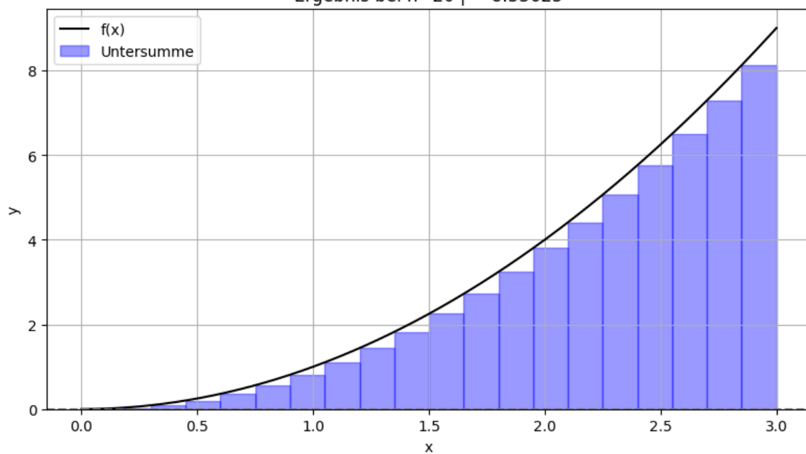
Numerische Integration mittels Untersumme Ergebnis bei n=20 \mid \approx 8.33625
