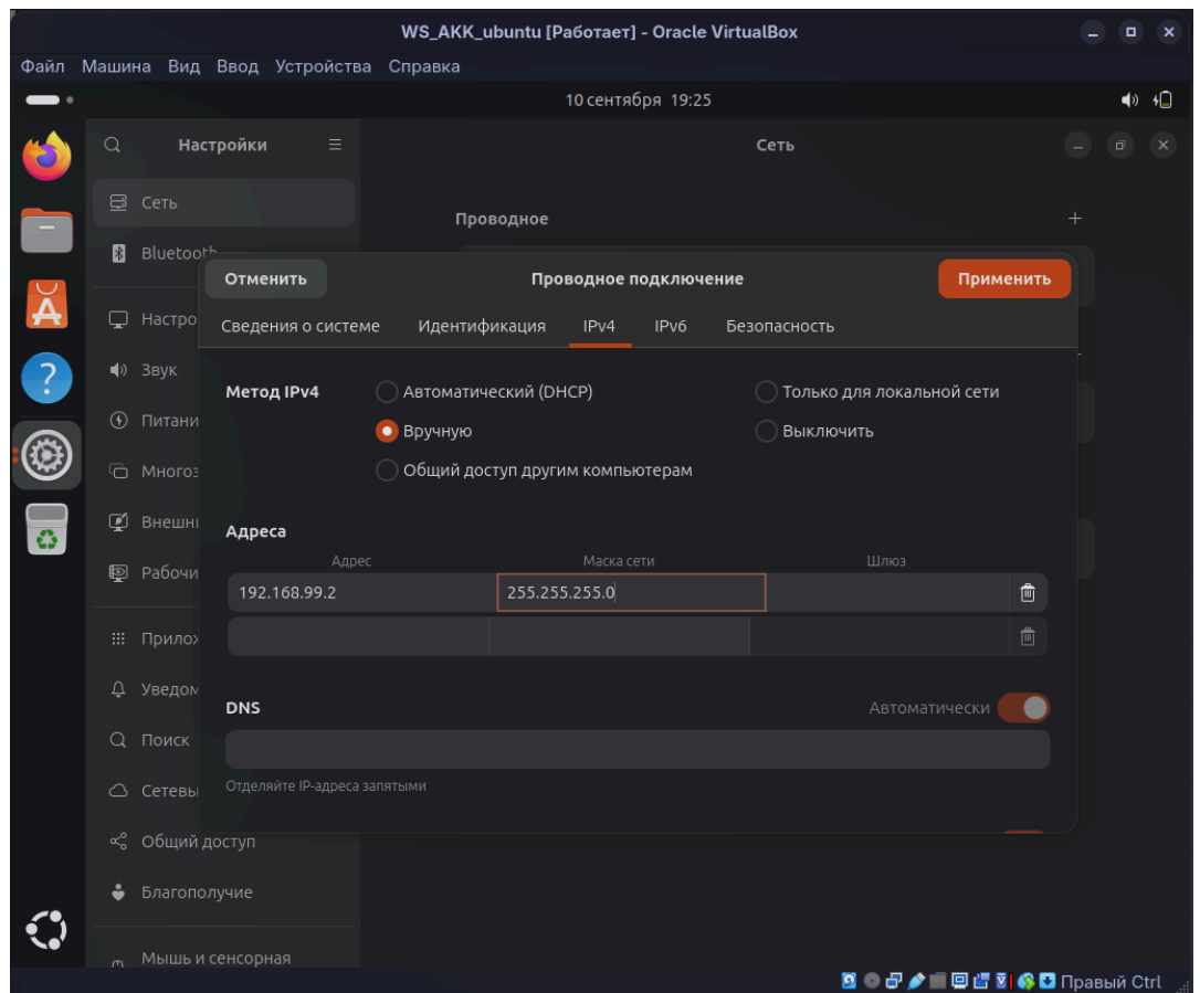
Рисунок 4 — IP-адрес Ubuntu
