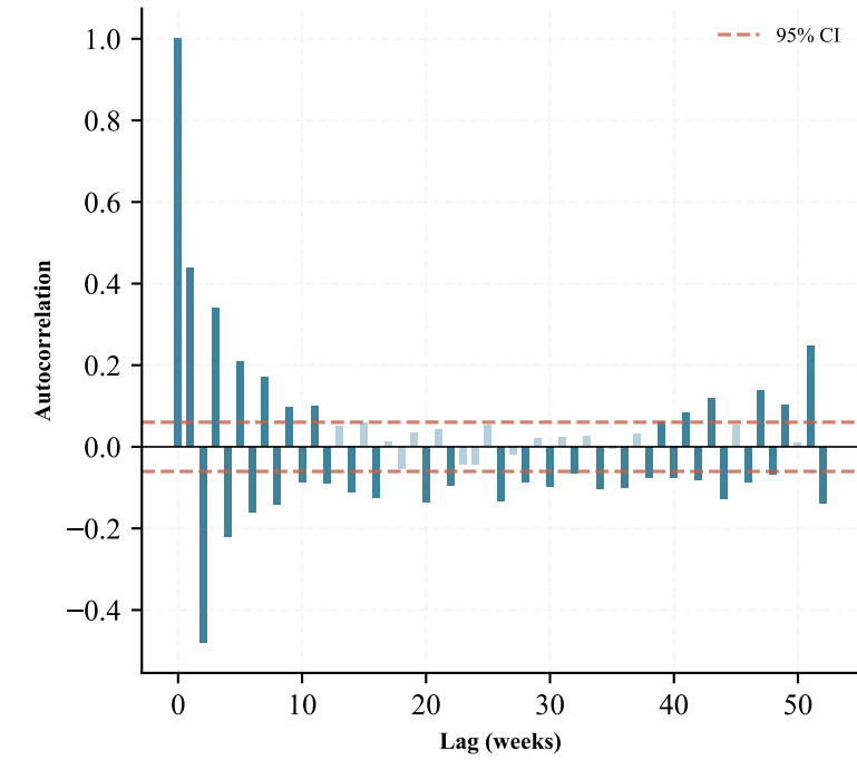
PACF (Y 1w)
