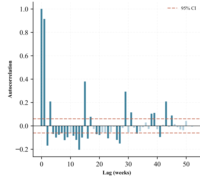
PACF (Y 3m)
