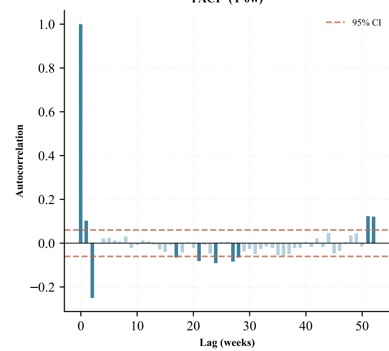
PACF (Y 0w)
