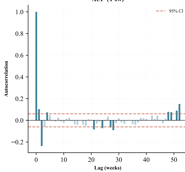
ACF (Y 0w)
