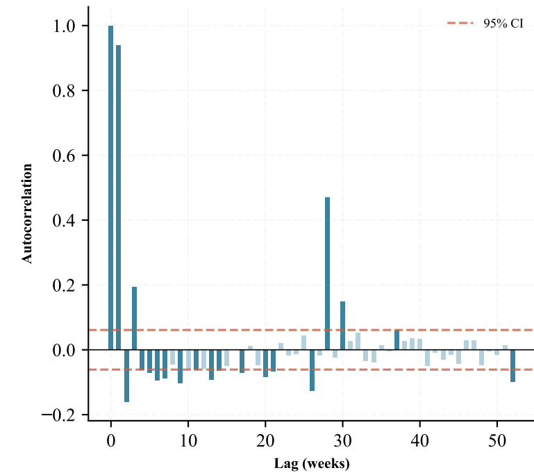
PACF (Y 6m)
