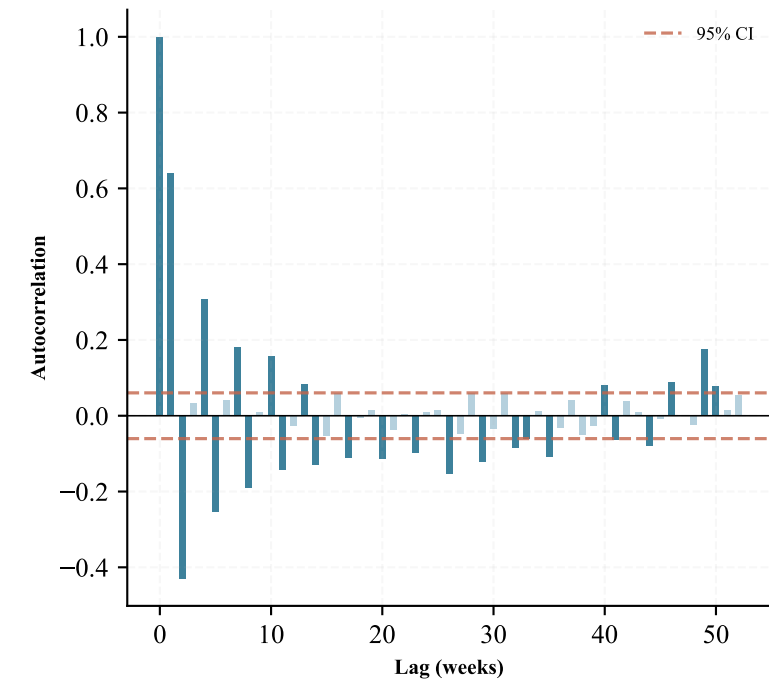
PACF (Y 2w)
