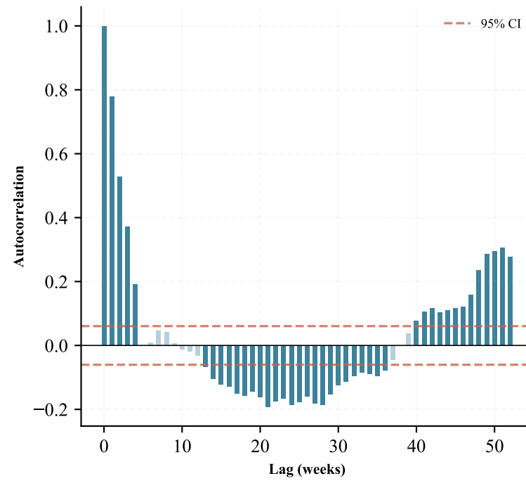
ACF (Y 1m)
