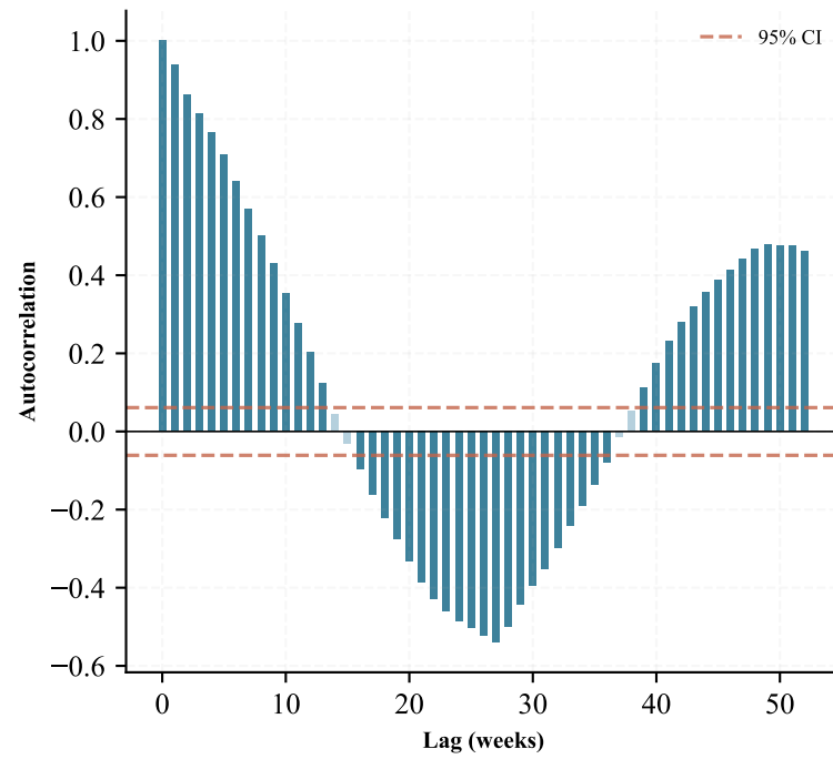
ACF (Y 6m)
