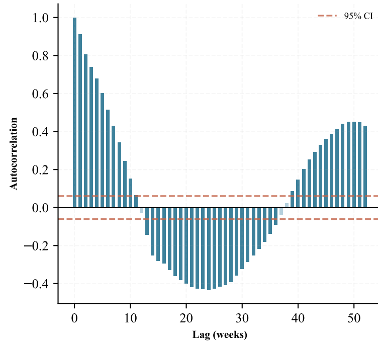
ACF (Y 3m)
