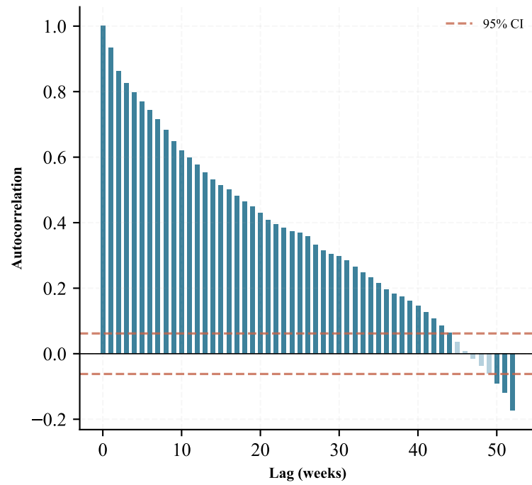
ACF (Y 12m)
