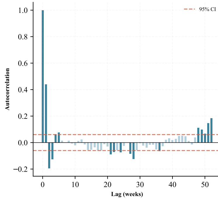
ACF (Y 1w)
