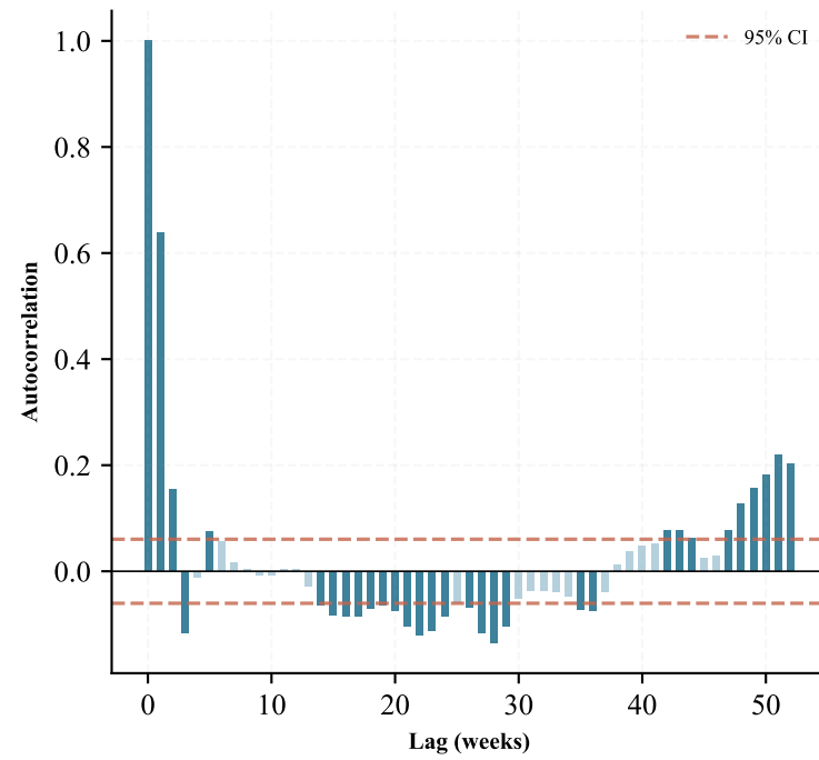
ACF (Y 2w)
