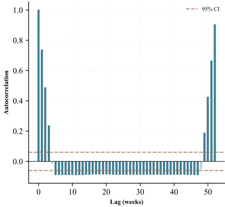
ACF (Month_04)
