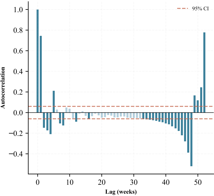
PACF (Month_06)
