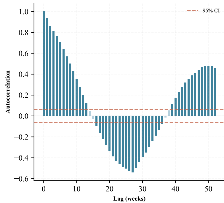
ACF (Y 6m)
