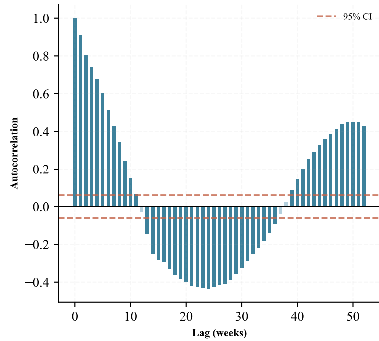
ACF (Y 3m)
