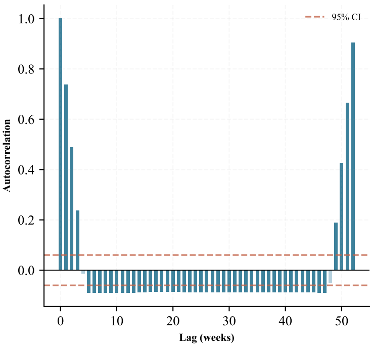
ACF (Month_04)
