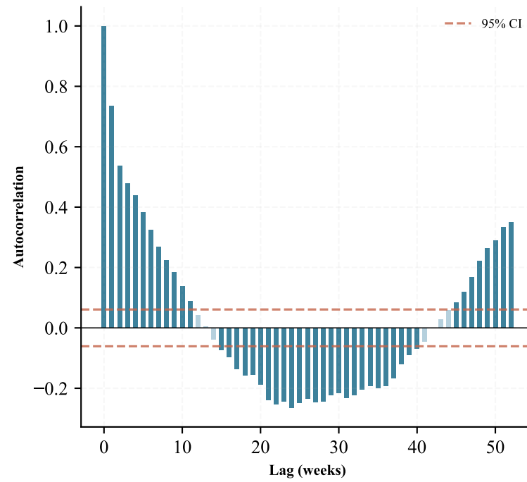
ACF (FWD 1m)
