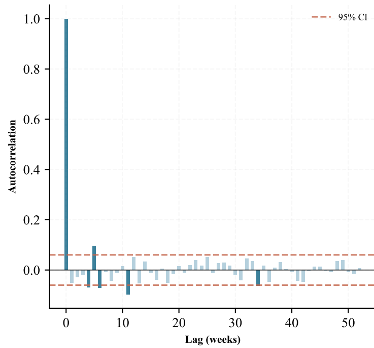
ACF ( \Delta EURNOK)
