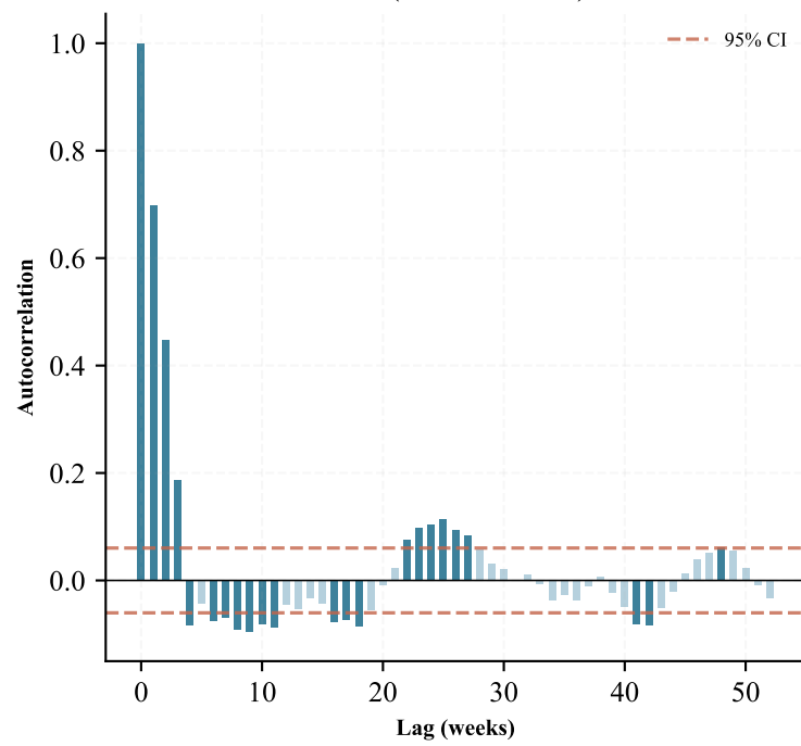
ACF ( \Delta EURNOK 1m)
