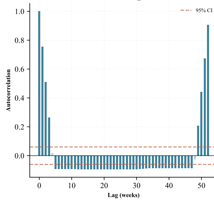
ACF (Month_08)
