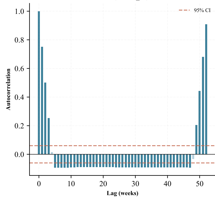
ACF (Month_01)
