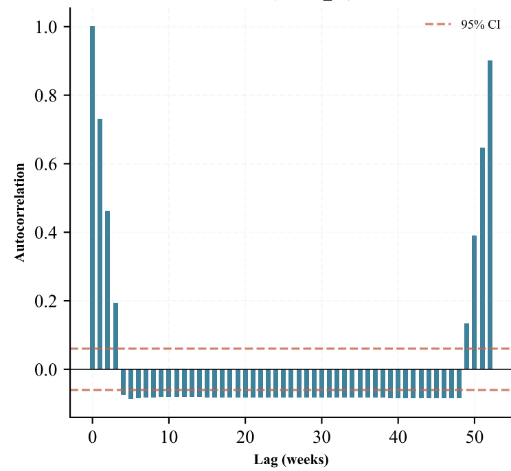
ACF (Month_02)
