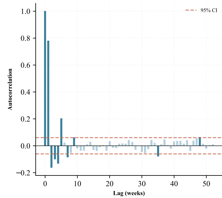
PACF (RVol 4w)
