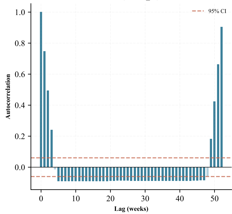
ACF (Month_11)
