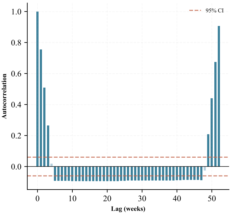
ACF (Month_10)
