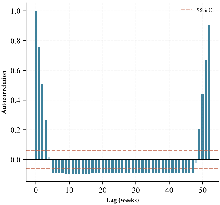
ACF (Month_05)
