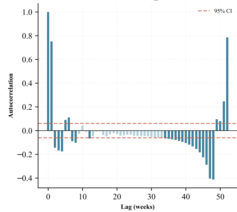
PACF (Month_01)
