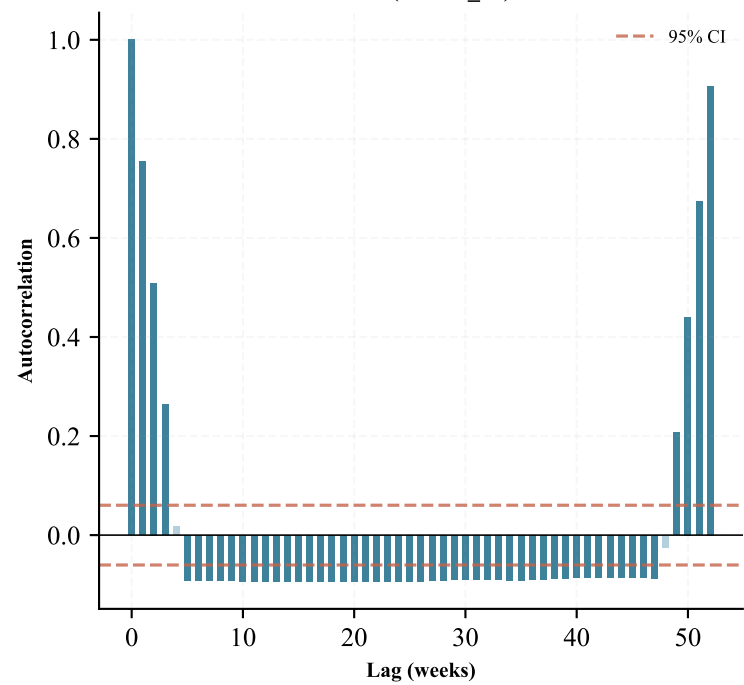
ACF (Month_07)
