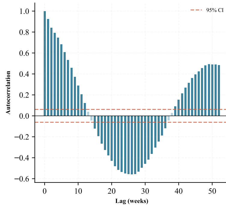
ACF (FWD 6m)
