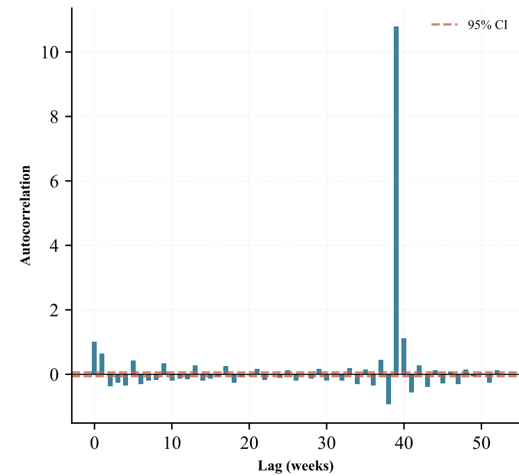
PACF (Acc 1m)
