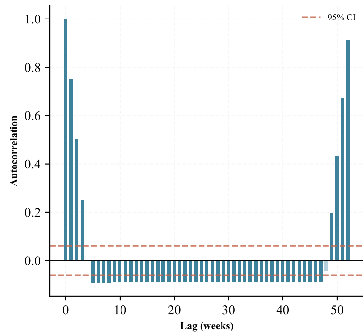
ACF (Month_03)
