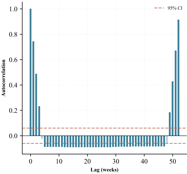
ACF (Month_09)
