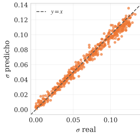
(b) Predicción de \sigma ( R^2=0.981 )
