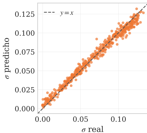
(b) Predicción de \sigma ( R^2=0.982 )
