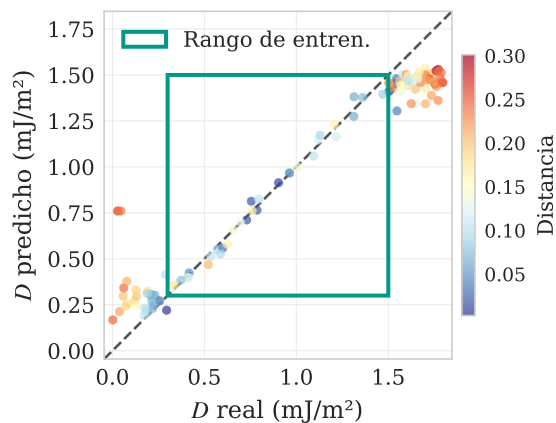
(a) Predicción de D ( R^2=0.903 )
