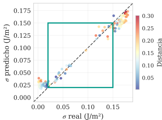
(b) Predicción de \sigma ( R^2=0.953 )
