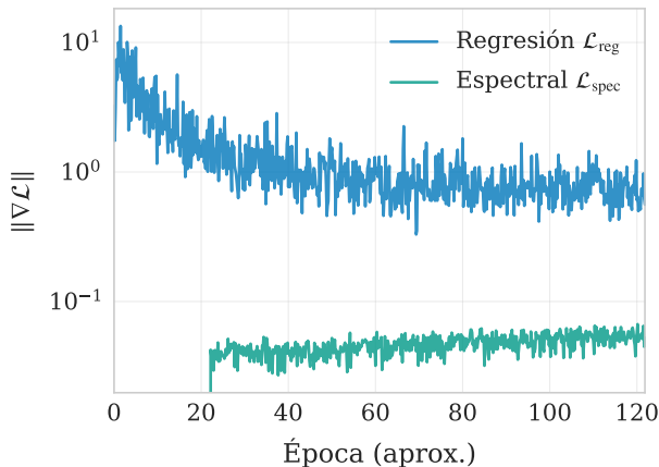
(a) Magnitud de gradientes
