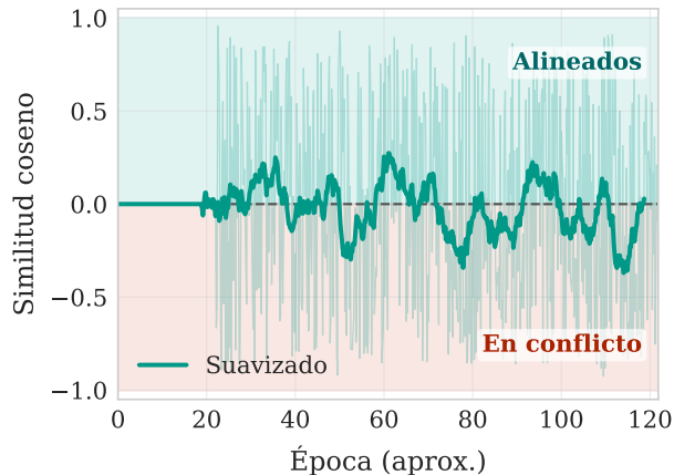
(b) Alineación \nabla \mathcal{L}_{\text{reg}} \leftrightarrow \nabla \mathcal{L}_{\text{spec}}
