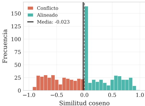
(d) Distribución de alineación (conflicto: 42.9%)
