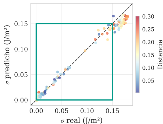
(b) Predicción de \sigma ( R^2=0.975 )
