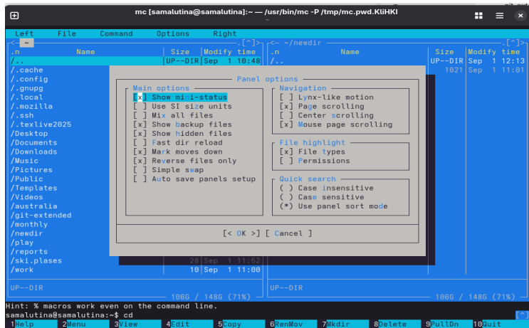
Рисунок 21: Настройки панелей
