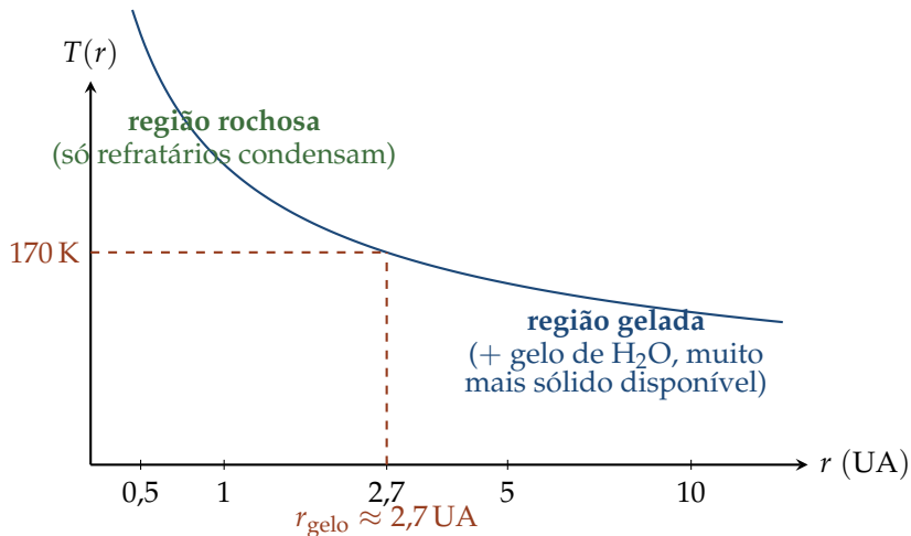
Figura 7.7: Perfil T(r) \propto r^{-1/2} [Equação (7.51), normalização MMSN] com a linha de gelo ( T = 170 \text{ K} , r_{\text{gelo}} \approx 2,7 \text{ UA} ) separando a região onde só refratários condensam da região onde o gelo de água também condensa.
