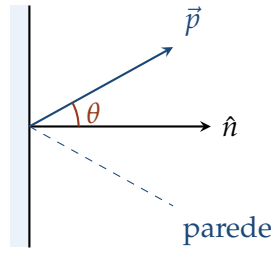
Figura 8.3: Geometria usada na dedução da pressão cinética: uma partícula de momento \vec{p} colide com a parede (normal \hat{n} ) fazendo um ângulo \theta com a normal; a reflexão especular transfere momento \Delta p = 2p \cos \theta para a parede.
