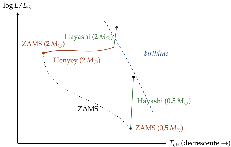
Figura 7.4: Evolução PMS de duas massas: para 0,5 M_\odot (verde), o traço de Hayashi domina toda a contração ( \sim 1,6 \times 10^8 anos até a ZAMS); para 2 M_\odot , um curto Hayashi é seguido de Henyey (laranja, L quase constante) até a ZAMS em apenas \sim 10^7 anos. A birthline tracejada marca onde protoestrelas se tornam visíveis (Seção 7.6).
