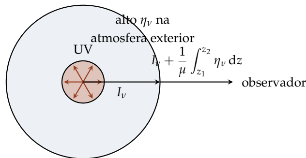
Figura 4.10: Estrutura estrela+nebulosa: a estrela central quente emite radiação UV que ioniza o gás circundante, produzindo alta emissividade \eta_v na camada externa (a nebulosa). O feixe I_v vindo do disco estelar central atravessa a nebulosa e chega ao observador somado à emissão acumulada ao longo do caminho, conforme a Equação (4.68).
