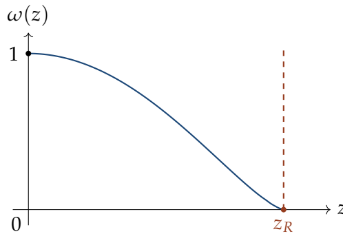
Figura 6.2: Comportamento esquemático da função de Lane–Emden \omega(z) : decresce monotonicamente a partir de \omega(0) = 1 no centro da estrela ( z = 0 ) até se anular no raio politrópico z = z_R (linha tracejada), que marca a superfície estelar.
