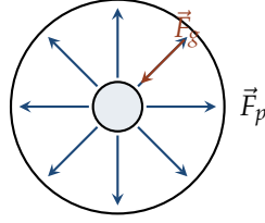
Figura 5.3: Estrela em equilíbrio hidrostático: a força de pressão \vec{F}_p (para fora, em cada direção) equilibra exatamente a força gravitacional \vec{F}_g (para dentro) em cada camada — F_g = F_p .
