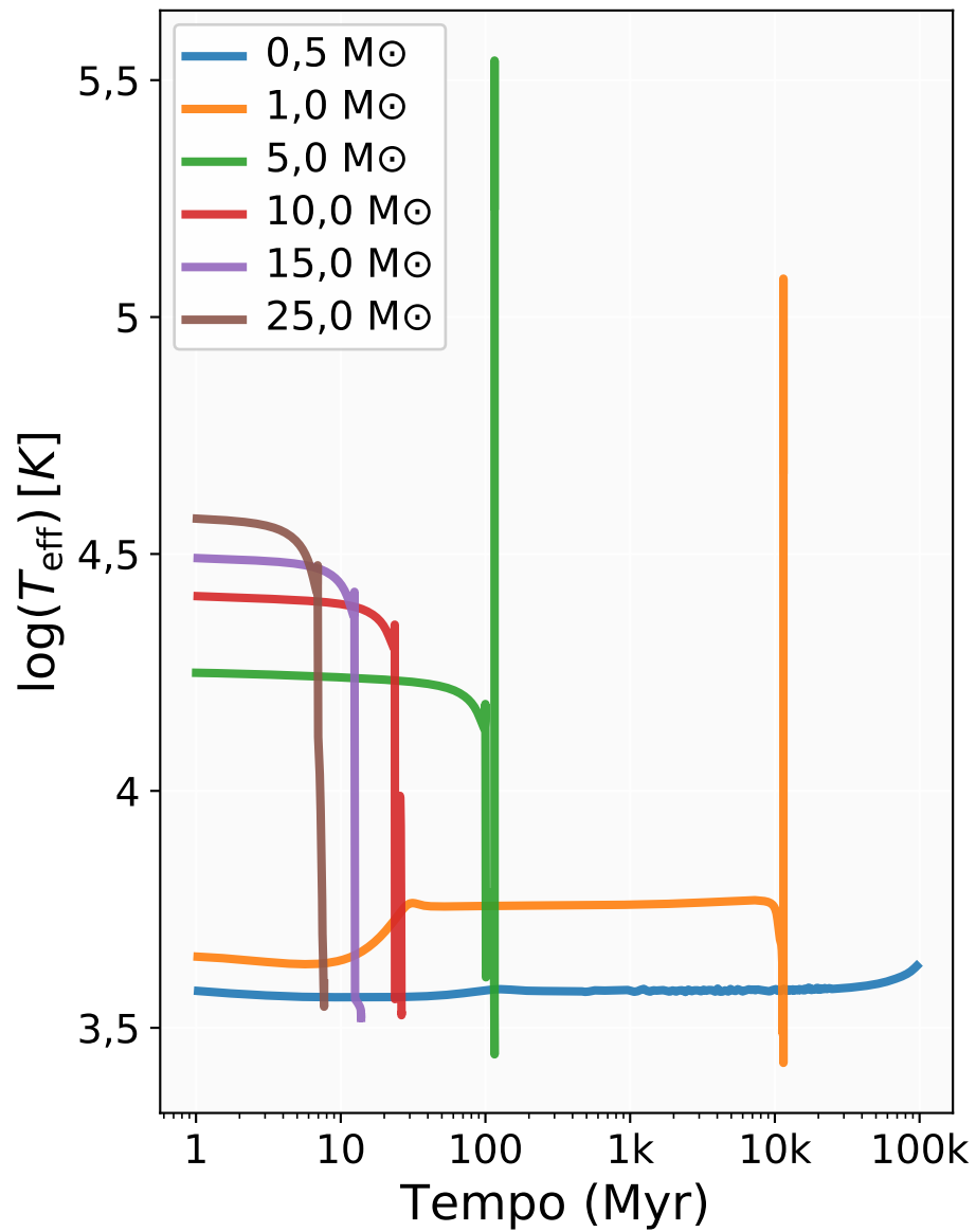
Figura 11.7: Temperatura efetiva em função do tempo para estrelas de 0,5 a 25 M_{\odot} , evidenciando a estabilidade térmica em baixas massas, o resfriamento pronunciado durante a fase de gigante e o aumento abrupto de temperatura nas etapas finais da evolução.
