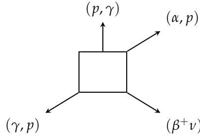
Figura 10.4: Esquema geral dos quatro tipos de transição que conectam espécies vizinhas na carta de nuclídeos: captura de próton, captura de partícula \alpha , fotodissociação com emissão de próton, e decaimento \beta^+ .
