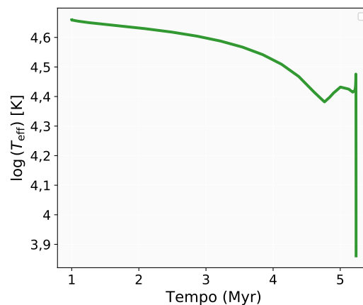
Figura 11.26: Diminuição da temperatura efetiva indicando expansão do envelope estelar.
