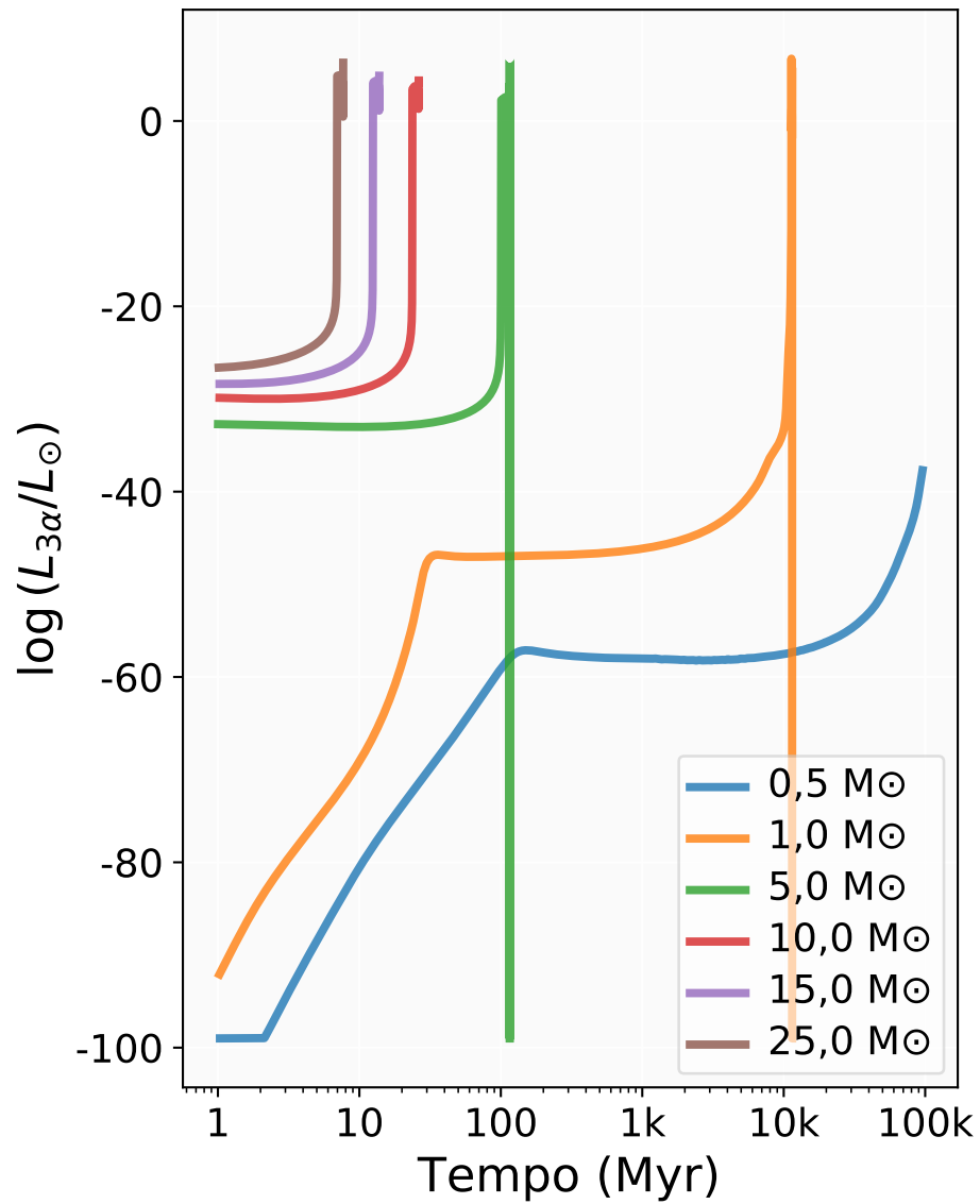
Figura 11.10: Variação temporal da luminosidade nuclear associada ao processo tripla- \alpha , mostrando sua ativação tardia em estrelas de baixa massa e sua rápida intensificação e curta duração em estrelas intermediárias e massivas durante a queima de hélio.
