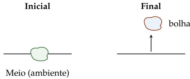
Figura 5.7: Esquema da bolha de gás: no instante inicial, ela está em equilíbrio com o meio (ambiente); no instante final, já subiu em relação à sua posição original. A denota o ambiente e B a bolha.
