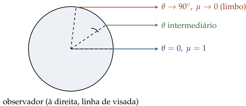
Figura 4.16: Escurecimento de limbo: em geometria plano-paralela, camadas mais externas e mais frias da atmosfera dominam a intensidade emergente quando o ângulo \theta entre a linha de visada e a normal local aumenta ( \mu = \cos \theta diminui) — ou seja, ao se observar cada vez mais perto da borda do disco estelar.
