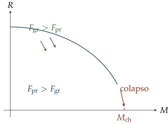
Figura 9.2: Relação massa-raio esquemática de anãs brancas: curva decrescente separando a região estável ( F_{pr} > F_{gr} , sustentada por degenerescência eletrônica) da região instável ( F_{gr} > F_{pr} ), com o colapso ocorrendo ao se aproximar da massa de Chandrasekhar, M_{ch} , no eixo horizontal.
