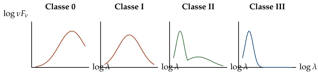
Figura 7.5: SEDs esquemáticas ( \log \nu F_{\nu} vs. \log \lambda ) da sequência Classe 0 → I → II → III: o pico se desloca de comprimentos de onda longos (envelope frio) para curtos (fotosfera), à medida que envelope e disco se dissipam — a mesma sequência de M_{\text{env}}/M_{\star} decrescente da caixa anterior.
