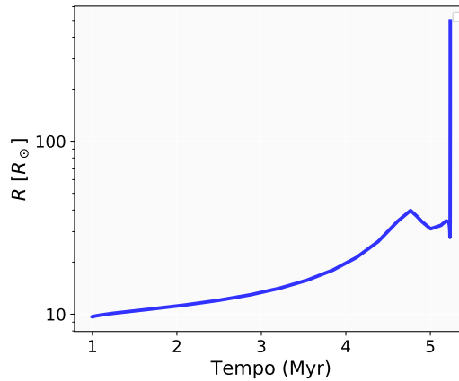
Figura 11.27: Crescimento exponencial do raio, atingindo quase 500 R_{\odot} .
