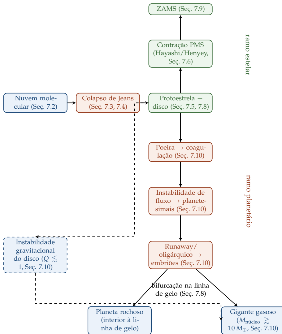
Figura 7.9: Fluxo resumindo o capítulo: do colapso de um núcleo pré-estelar até a bifurcação entre o ramo estelar (contração PMS até a ZAMS) e o planetário (poeira a planetas rochosos ou gigantes gasosos, com a linha de gelo determinando o destino). O canal tracejado (instabilidade gravitacional do disco) contorna a física colisional do ramo planetário principal — a única etapa genuinamente análoga à física estelar (Seção 7.10).
