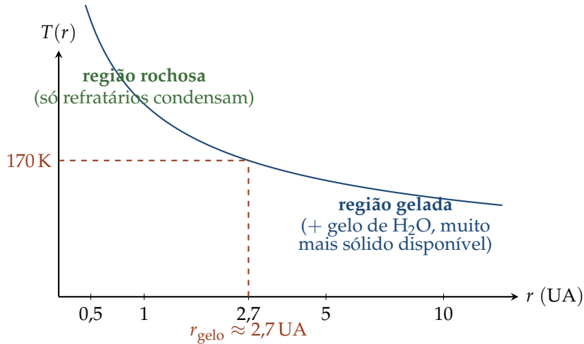
Figura 7.7: Perfil T(r) \propto r^{-1/2} [Equação (7.51), normalização MMSN] com a linha de gelo ( T = 170 K, r_{\text{gelo}} \approx 2,7 UA) separando a região onde só refratários condensam da região onde o gelo de água também condensa.
