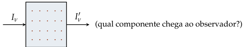
Figura 4.6: Feixe luminoso atravessando um gás qualquer. As interações eletromagnéticas com o meio modificam I_\nu , resultando em I'_\nu .
