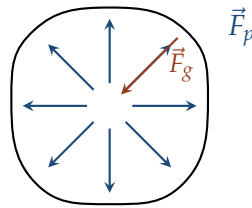
Figura 5.2: Nuvem de gás autogravitante: quando a força gravitacional \vec{F}_g supera a força de pressão do gás \vec{F}_p , a nuvem colapsa — o início da instabilidade de Jeans.
