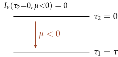
Figura 4.14: Caso \mu < 0 : sem radiação externa incidente sobre a estrela, I_\nu(\tau_2 = 0, \mu < 0) = 0 é a condição de contorno natural no topo da atmosfera.
