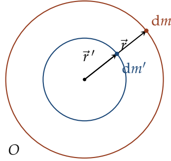
Figura 6.1: Duas cascas esféricas concêntricas, de elementos de massa dm (raio r ) e dm' (raio r' ), usadas na dedução do potencial gravitacional em simetria esférica.
