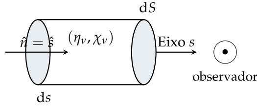
Figura 4.7: Cilindro de gás com coeficientes de opacidade \chi_\nu e emissividade \eta_\nu , atravessado ao longo do eixo s .
