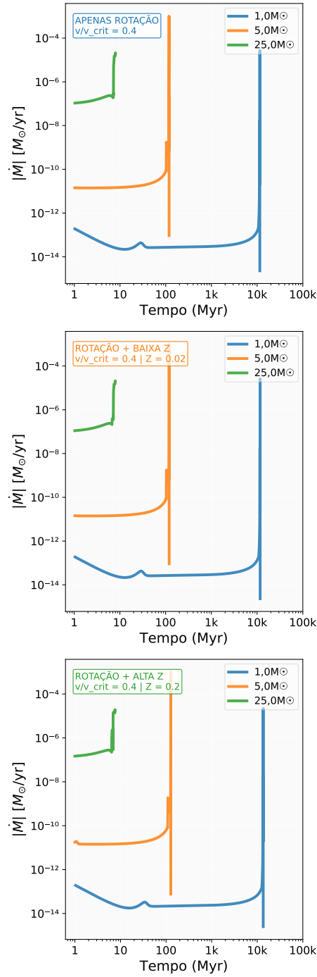
Figura 11.17: Comparação da perda de massa ao longo do tempo para diferentes configurações de rotação e metalicidade, evidenciando o papel combinado da opacidade e do achatamento rotacional na eficiência dos ventos estelares.
