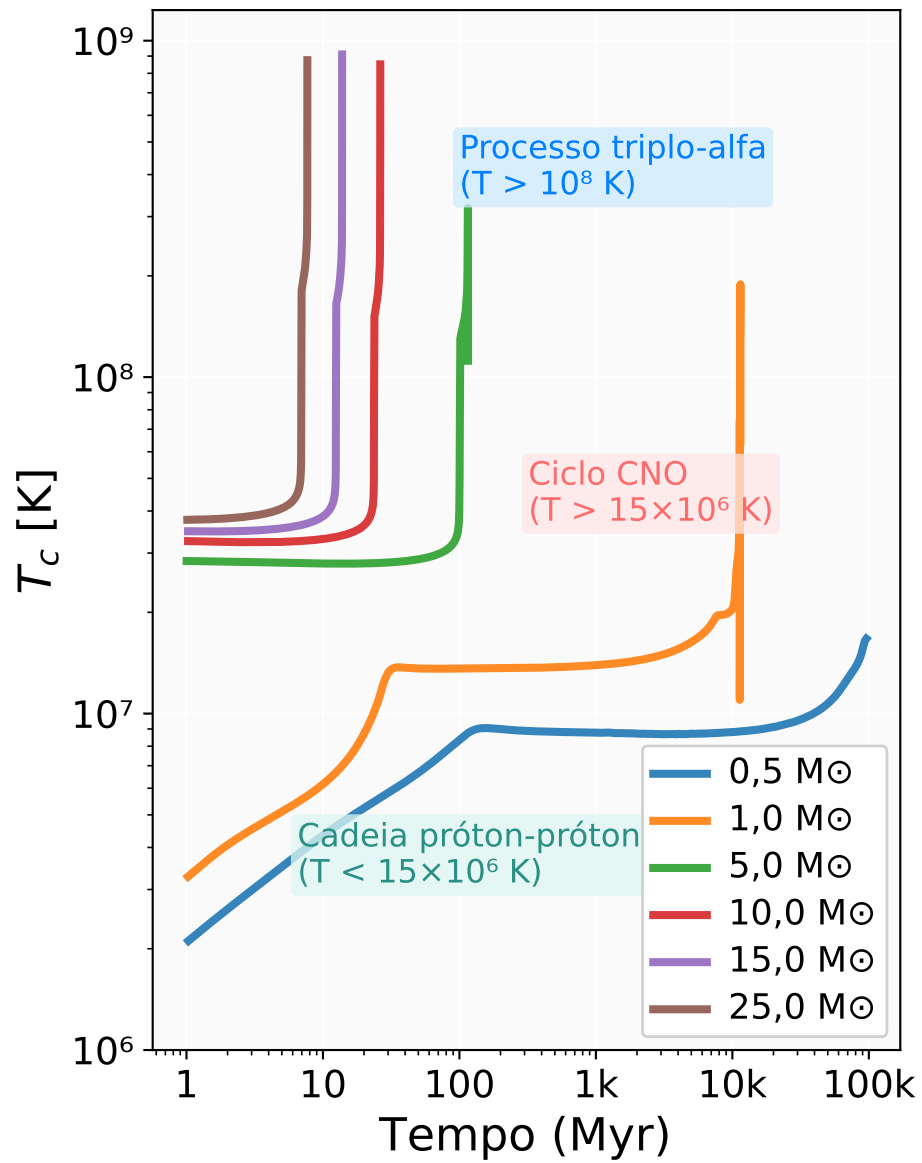
Figura 11.11: Evolução temporal da temperatura central para estrelas de diferentes massas, desde a sequência principal até as fases avançadas de queima nuclear. A progressão crescente de T_c reflete a contração gravitacional do núcleo à medida que os combustíveis são esgotados, revelando claramente as transições entre os regimes de fusão dominantes para cada faixa de massa.
