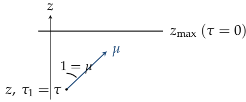
Figura 4.11: Feixe emergente com \mu = 1 : percurso de um ponto qualquer z (profundidade \tau_1 = \tau ) até o topo da atmosfera z_{\max} (\tau = 0) .
