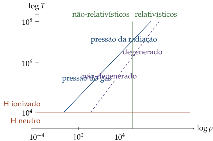
Figura 8.4: Diagrama densidade–temperatura esquemático mostrando as principais fronteiras discutidas neste capítulo: dominância de pressão de radiação vs. pressão do gás (linha sólida diagonal); gás não-degenerado vs. degenerado (linha tracejada diagonal); hidrogênio neutro vs. ionizado (linha horizontal perto de T \sim 10^4 K); e elétrons não-relativísticos vs. relativísticos (linha vertical em alta densidade).
