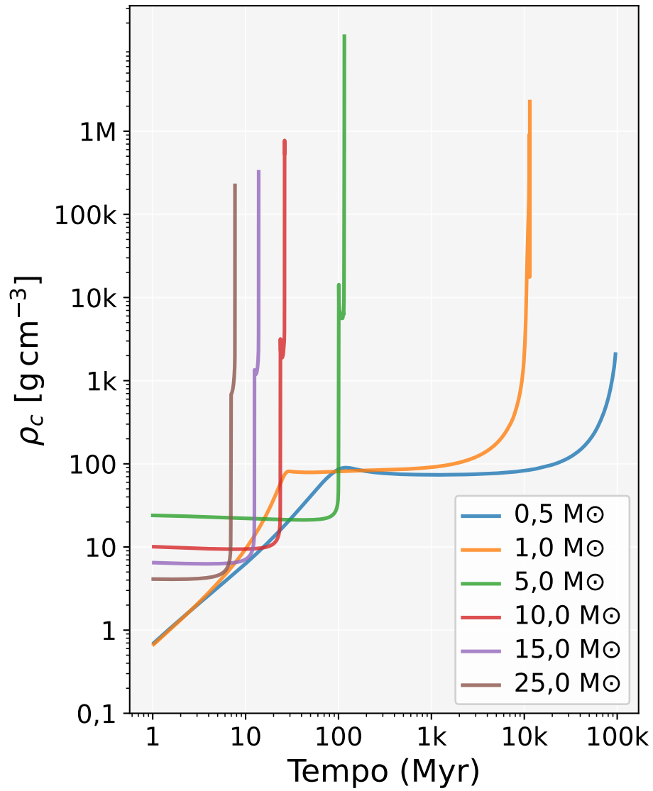
Figura 11.12: Evolução temporal da densidade central para estrelas de diferentes massas. O crescimento de \rho_c reflete a contração gravitacional do núcleo e a transição entre regimes de suporte por pressão térmica, degenerescência eletrônica e, em estrelas massivas, pressão de radiação.
