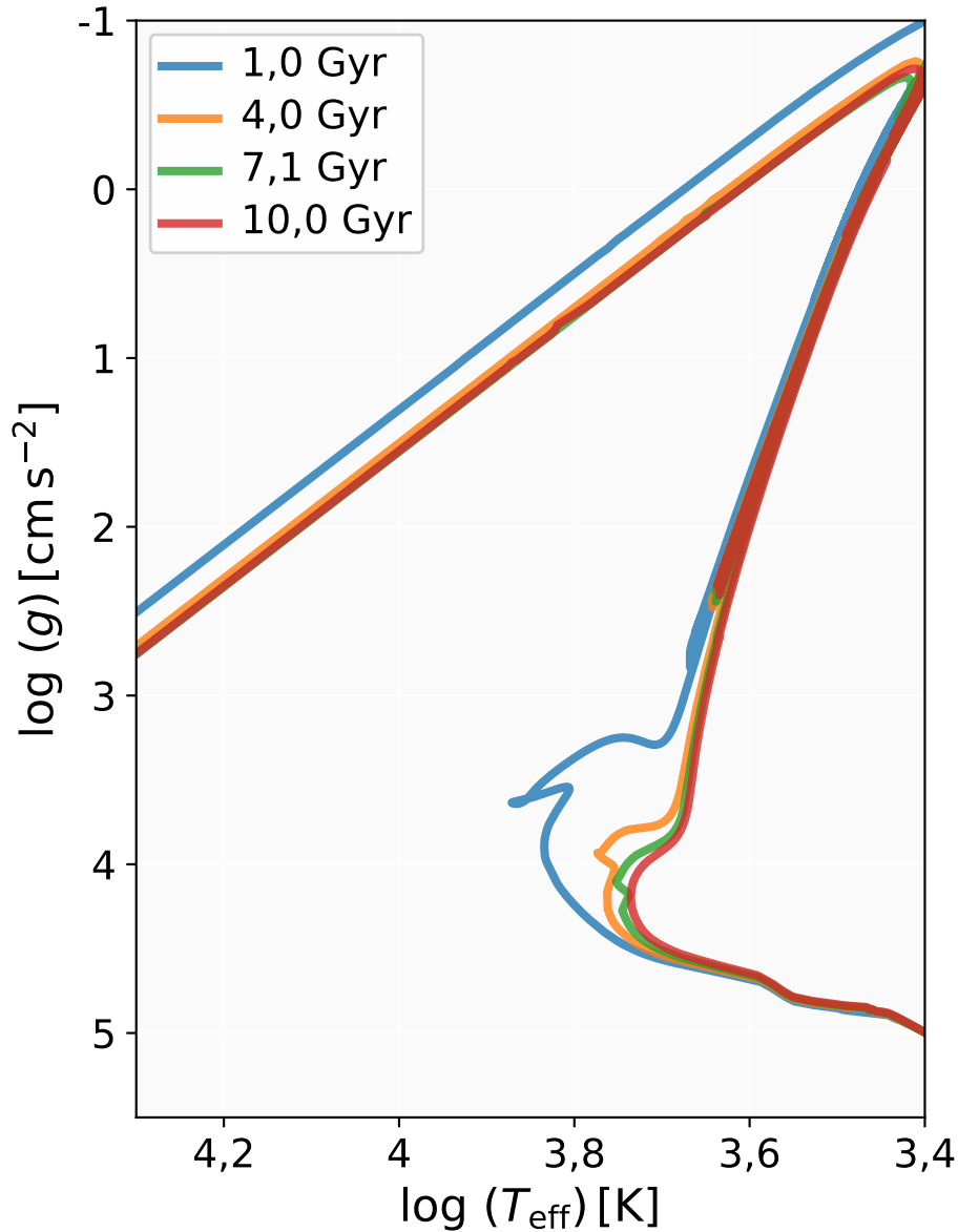
Figura 11.23: Isócronas para [Fe/H] = +0,5 . A alta metalicidade produz o maior deslocamento para baixas temperaturas e o ramo das gigantes mais expandido entre todos os casos analisados.
