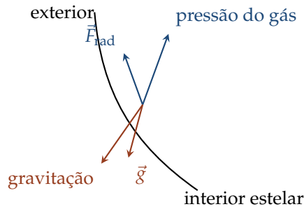
Figura 4.17: Equilíbrio de forças em um elemento de gás na estrela: a pressão do gás e a força radiativa \vec{F}_{\text{rad}} (para fora) equilibram a força gravitacional \vec{g} (para dentro). No limite de Eddington, a força radiativa sozinha iguala a força gravitacional.
