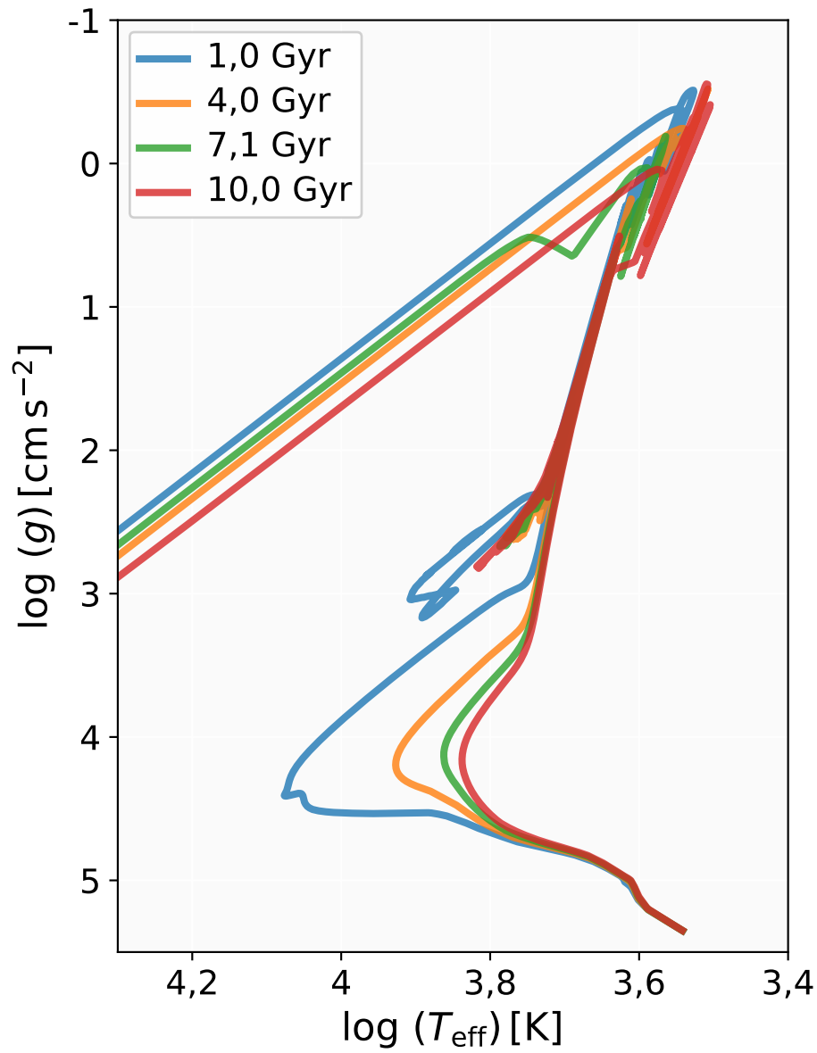
Figura 11.20: Isócronas no Diagrama de Kiel para [Fe/H] = -2 e idades de 1, 4, 7 e 10 Gyr. A baixa opacidade desloca a sequência principal para temperaturas mais altas e comprime o ramo das gigantes.
