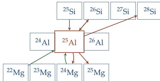
Figura 10.3: Fragmento da carta de nuclídeos centrado em ^{25}\text{Al} . Setas verdes indicam reações que geram ^{25}\text{Al} ; setas vermelhas indicam reações que o destroem.
