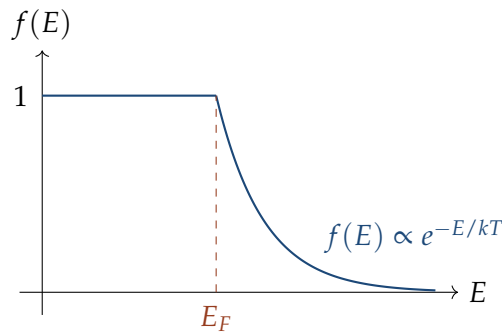
Figura 8.1: Probabilidade de ocupação f(E) de um estado de energia E para um gás de elétrons. Em T = 0 (degenerescência total), f(E) é um patamar em 1 até E_F e cai abruptamente a 0; a temperaturas finitas, a distribuição decai suavemente como e^{-E/kT} acima de E_F .
