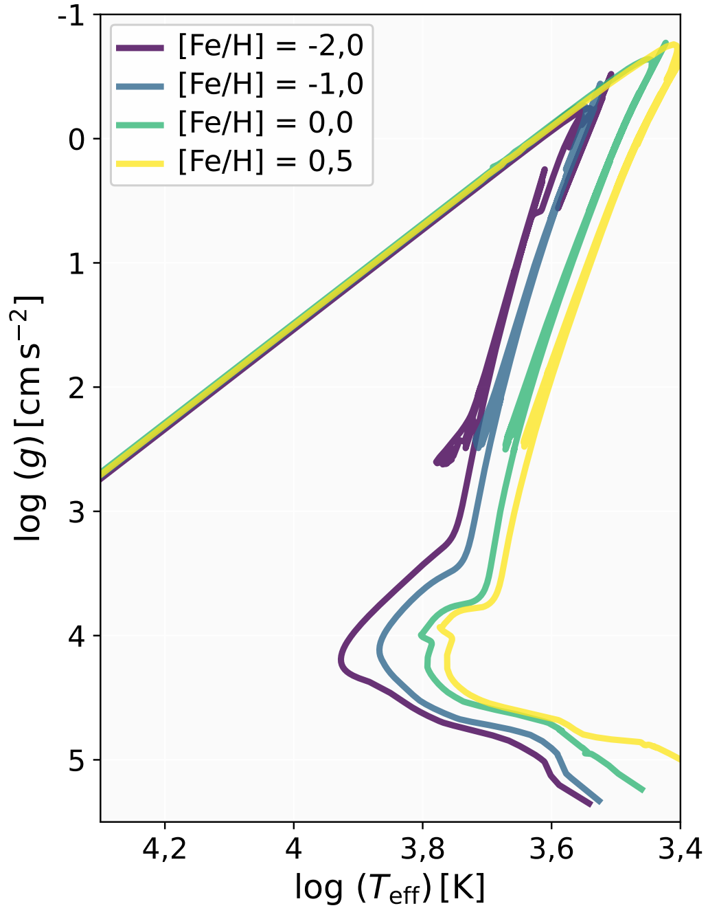
Figura 11.19: Diagrama de Kiel para isócronas de 4 Gyr com diferentes metalicidades. As curvas demonstram o deslocamento da sequência principal em função do conteúdo metálico.
