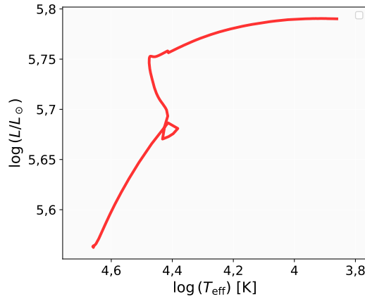
Figura 11.24: Trajetória evolutiva da estrela de 50 M_{\odot} no diagrama HR. A estrela inicia quente e luminosa na sequência principal e evolui para a região das supergigantes.
