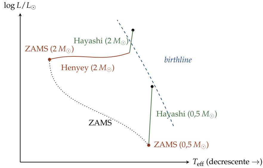
Figura 7.4: Evolução PMS de duas massas: para 0,5 M_{\odot} (verde), o traço de Hayashi domina toda a contração ( \sim 1,6 \times 10^8 anos até a ZAMS); para 2 M_{\odot} , um curto Hayashi é seguido de Henyey (laranja, L quase constante) até a ZAMS em apenas \sim 10^7 anos. A birthline tracejada marca onde protoestrelas se tornam visíveis (Seção 7.6).
