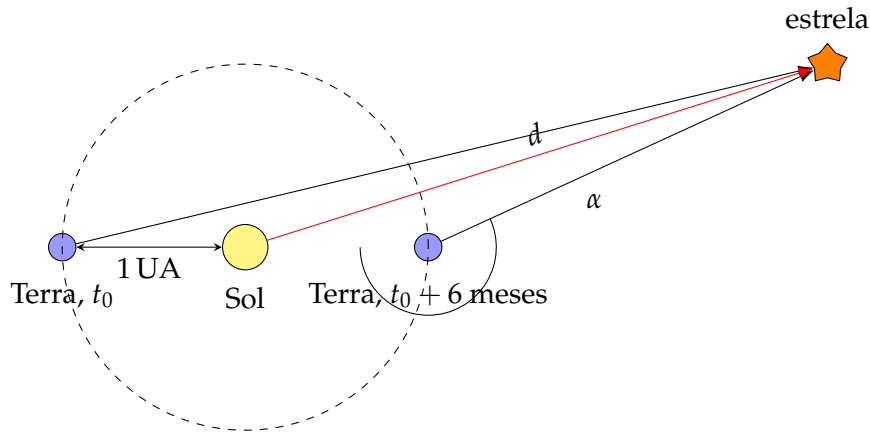
Figura 1.1: Geometria da paralaxe estelar: a Terra ocupa posições opostas de sua órbita com seis meses de intervalo, o que permite medir o pequeno deslocamento angular \alpha da estrela em relação ao fundo de estrelas mais distantes.
