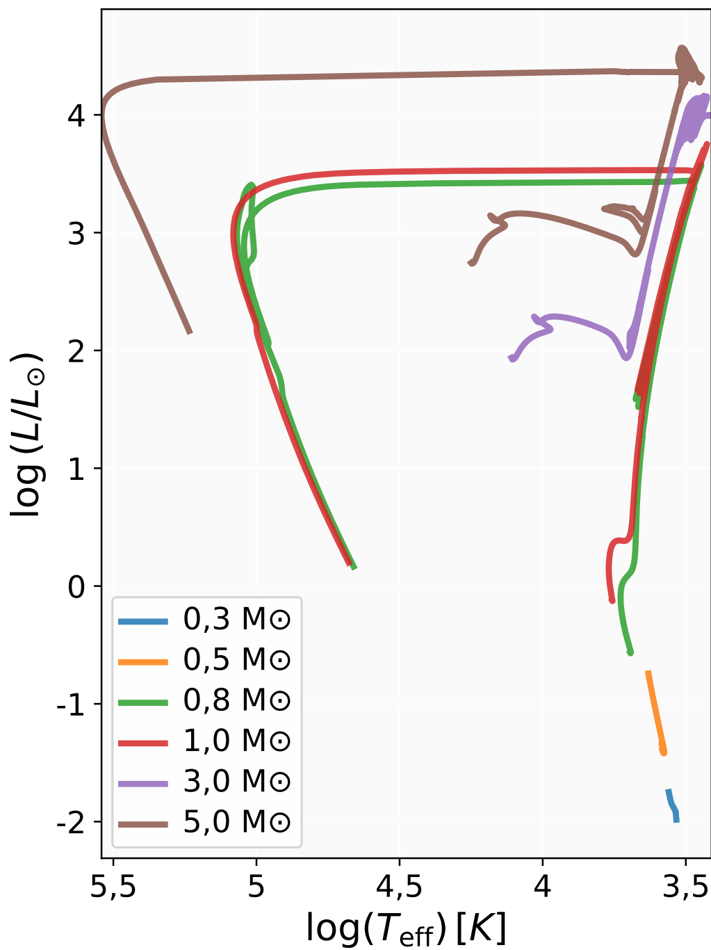
Figura 11.1: Diagrama HR para estrelas de baixa massa ( 0,3\text{--}5 M_\odot ).
