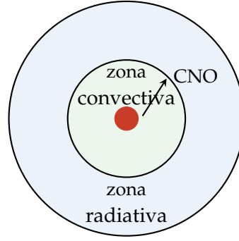
Figura 5.9: Estrutura de zonas de transporte de energia em uma estrela massiva (esquemático, fora de escala): núcleo com geração de energia via ciclo CNO, zona convectiva interna (envolvendo o núcleo) e zona radiativa externa — a configuração oposta à do Sol (Figura 5.6).
