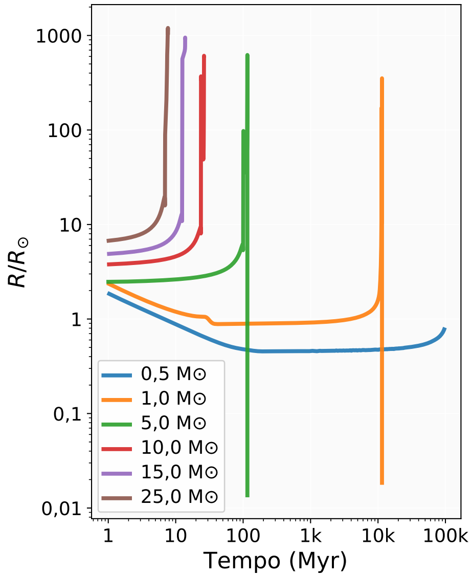
Figura 11.5: Evolução temporal do raio para estrelas entre 0,5 e 25 M_{\odot} , evidenciando a forte dependência do raio com a massa inicial e a expansão pronunciada nas fases pós-sequência principal.
