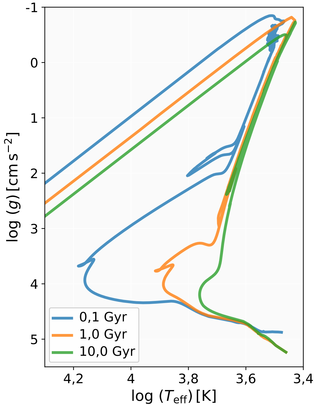
Figura 11.18: Diagrama de Kiel ( \log g versus \log T_{\text{eff}} ) mostrando isócronas para metalicidade solar em três idades representativas: 0,1, 1 e 10 Gyr. As curvas destacam a evolução da sequência principal, o deslocamento do ponto de turn-off e o desenvolvimento do ramo de gigantes vermelhas ao longo do tempo.
