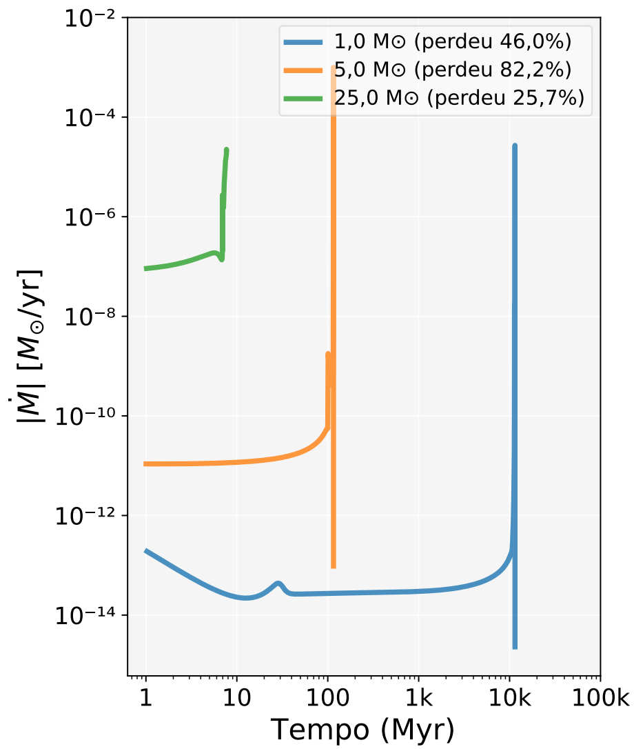
Figura 11.16: Principais fases evolutivas responsáveis pela perda de massa ao longo do tempo para diferentes massas estelares.
