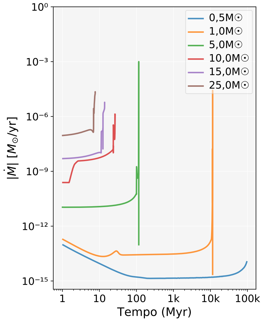
Figura 11.15: Evolução temporal da taxa de perda de massa para estrelas de diferentes massas, destacando os episódios associados a ventos estelares, pulsos térmicos e fases de gigante/supergigante.
