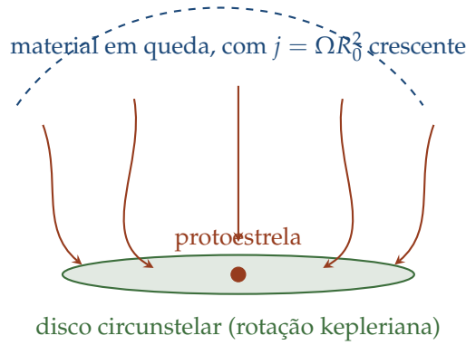
Figura 7.3: Formação do disco por deposição de material com j crescente: cada trajetória de infall conserva seu j e se deposita no raio centrífugo correspondente [Equação (7.29)] — material de baixo j cai quase direto sobre a protoestrela, o de alto j deposita-se em raios maiores, construindo um disco fino em rotação kepleriana.
