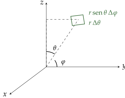
Figura 4.1: Elemento de ângulo sólido em coordenadas esféricas. A área da esfera de raio r limitada por (\theta, \theta + \Delta\theta) e (\varphi, \varphi + \Delta\varphi) é r^2 \sin \theta \Delta\theta \Delta\varphi , de modo que o ângulo sólido correspondente é \Delta\Omega = \sin \theta \Delta\theta \Delta\varphi .
