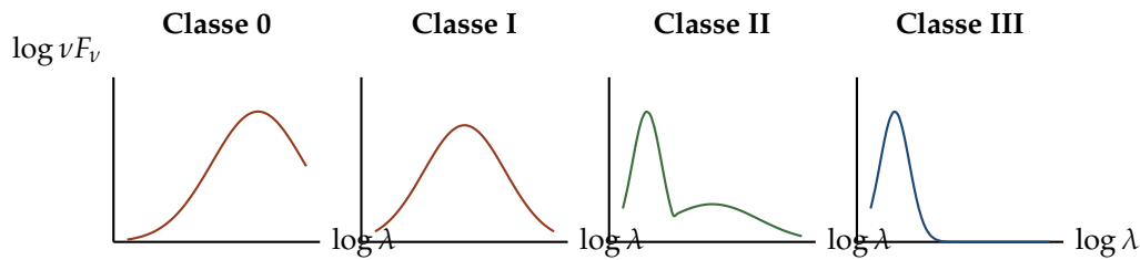
Figura 7.5: SEDs esquemáticas ( \log \nu F_{\nu} vs. \log \lambda ) da sequência Classe 0 \rightarrow I \rightarrow II \rightarrow III: o pico se desloca de comprimentos de onda longos (envelope frio) para curtos (fotosfera), à medida que envelope e disco se dissipam — a mesma sequência de M_{\text{env}}/M_* decrescente da caixa anterior.
