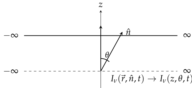
Figura 4.3: Geometria plano-paralela: a atmosfera é tratada como camadas horizontais semi-infinitas, de modo que I_\nu passa a depender apenas da profundidade z e do ângulo \theta em relação à normal.
