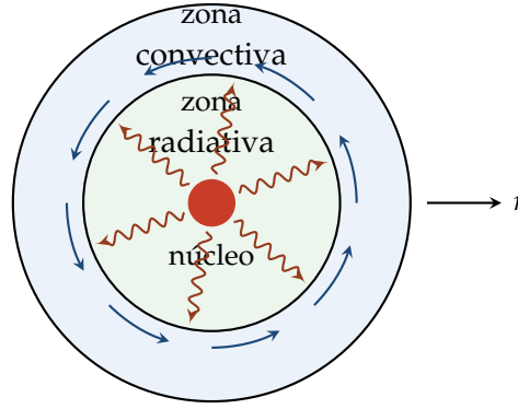
Figura 5.6: Estrutura de zonas de transporte de energia em uma estrela do tipo solar (esquemático, fora de escala): núcleo, zona radiativa (setas onduladas indicam fótons se difundindo lentamente para fora) e zona convectiva (setas curvas indicam células de convecção). Em estrelas do tipo solar, a zona radiativa domina os \approx 70\% internos do raio estelar, e a zona convectiva os \approx 30\% externos — mas, devido à forte queda de densidade em direção à superfície, a zona convectiva contém apenas \approx 2\% da massa da estrela.
