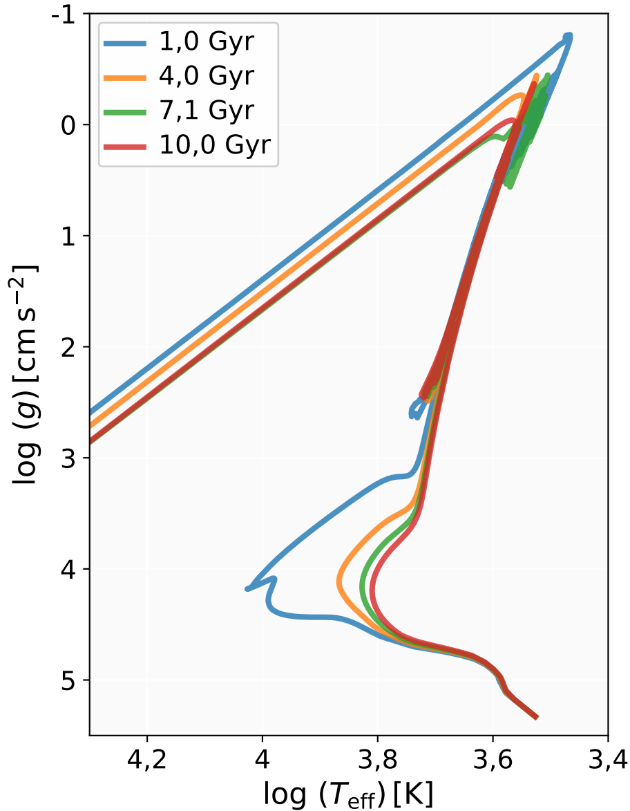
Figura 11.21: Isócronas para [Fe/H] = -1 . O aumento moderado da opacidade em relação a [Fe/H] = -2 desloca as curvas para temperaturas mais baixas e expande o ramo das gigantes.
