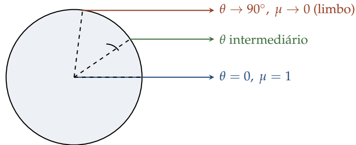
Figura 4.16: Escurecimento de limbo: em geometria plano-paralela, camadas mais externas e mais frias da atmosfera dominam a intensidade emergente quando o ângulo \theta entre a linha de visada e a normal local aumenta ( \mu = \cos \theta diminui) — ou seja, ao se observar cada vez mais perto da borda do disco estelar.
