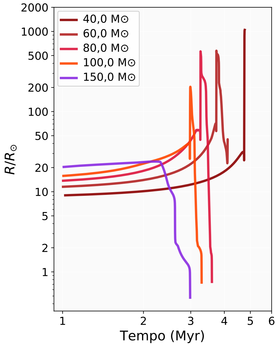
Figura 11.6: Evolução do raio para estrelas muito massivas (40–150 M_{\odot} ). O gráfico destaca a supressão da expansão em massas elevadas devido à pressão de radiação e às intensas perdas de massa por ventos estelares.
