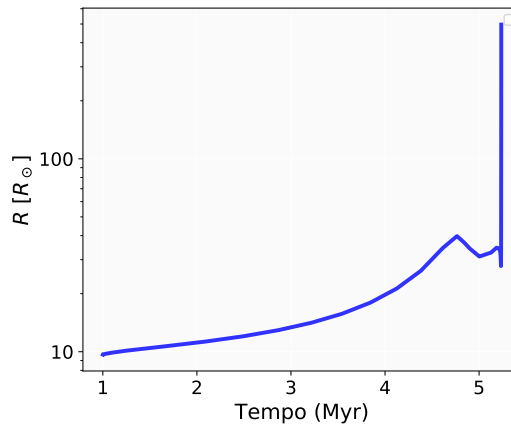
Figura 11.27: Crescimento exponencial do raio, atingindo quase 500 R_{\odot} .
