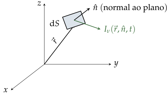
Figura 4.2: Feixe luminoso atravessando um elemento de área dS , com normal \hat{n} .
