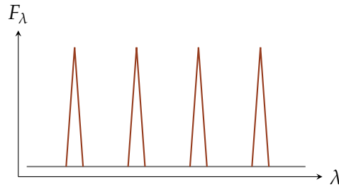
Figura 4.9: Espectro observado de uma nebulosa planetária: um contínuo fraco (a luz estelar central, atenuada pela distância) somado a linhas de emissão intensas e estreitas, produzidas pela recombinação de fótons no gás ionizado da nebulosa circundante.
