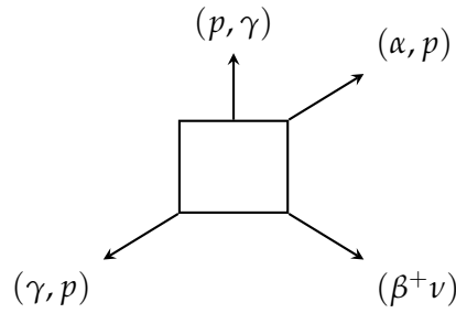
Figura 10.4: Esquema geral dos quatro tipos de transição que conectam espécies vizinhas na carta de núclídeos: captura de próton, captura de partícula \alpha , fotodissociação com emissão de próton, e decaimento \beta^+ .
