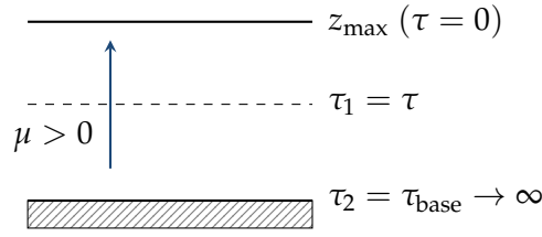
Figura 4.13: Caso \mu > 0 : o feixe se propaga de \tau_2 \rightarrow \infty (interior) até \tau_1 = \tau , em direção à superfície.
