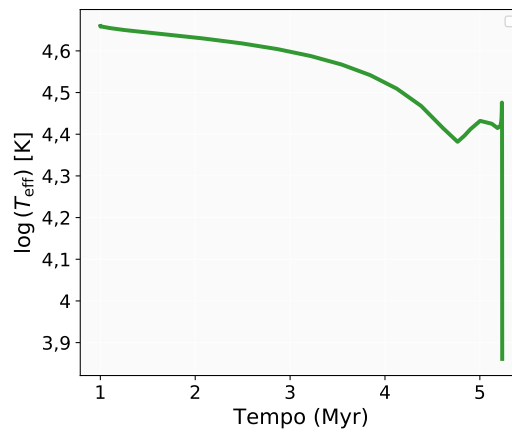
Figura 11.26: Diminuição da temperatura efetiva indicando expansão do envelope estelar.
