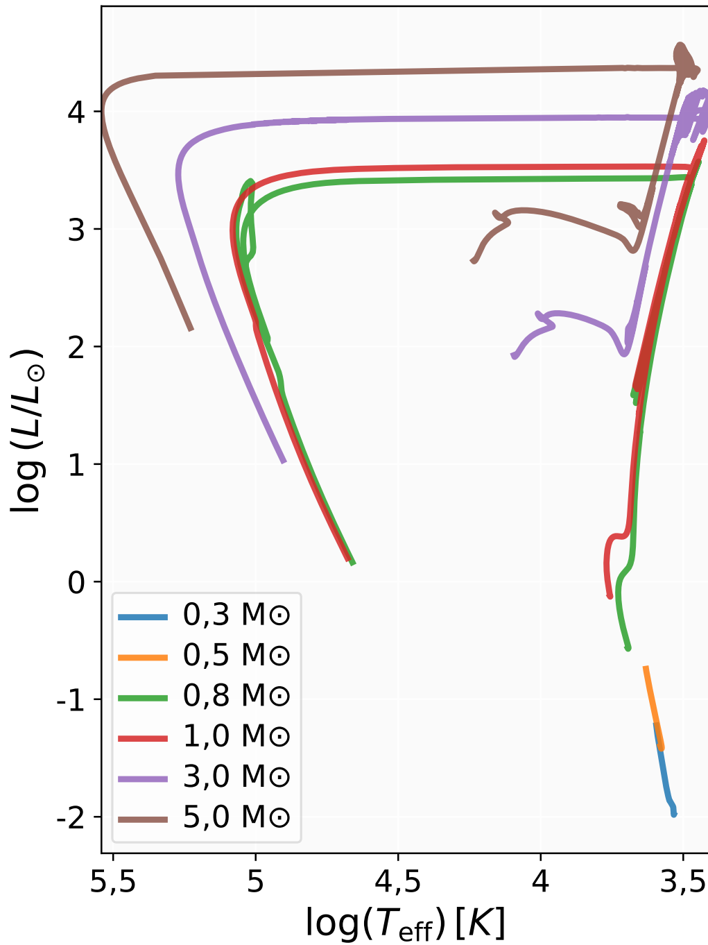
Figura 11.3: Diagrama HR para estrelas de baixa massa ( 0,3\text{--}5 M_{\odot} ) com rotação inicial v/v_{\text{crit}} = 0,4 . Comparado com a Figura 11.1, observa-se um deslocamento para temperaturas efetivas menores, acompanhado de ajustes na luminosidade, devido aos efeitos da mistura rotacional e ao escurecimento gravitacional.
