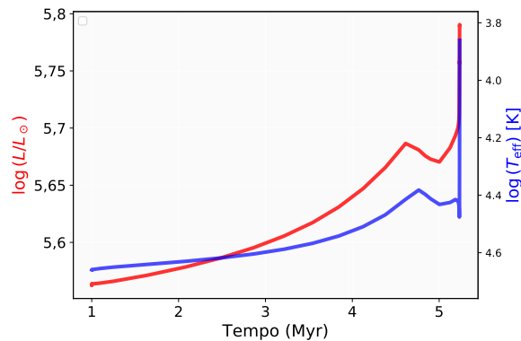
Figura 11.29: Comparação temporal entre luminosidade e temperatura, mostrando a diminuição da temperatura acompanhada de aumento na luminosidade.
