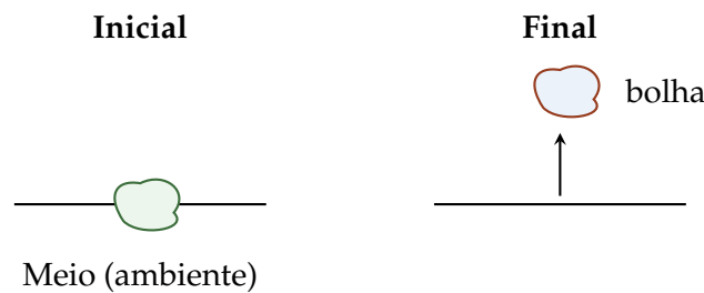
Figura 5.7: Esquema da bolha de gás: no instante inicial, ela está em equilíbrio com o meio (ambiente); no instante final, já subiu em relação à sua posição original. A denota o ambiente e B a bolha.
