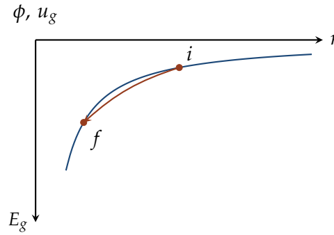
Figura 5.5: Trajetória de contração no plano (\phi, u_g) (ou, equivalentemente, E_g ) versus r : à medida que o raio diminui do estado inicial i para o final f , a energia potencial gravitacional torna-se mais negativa (a curva segue \propto -1/r ).
