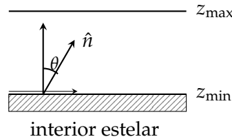
Figura 4.5: Profundidade de uma atmosfera plano-paralela, delimitada entre z_{\min} (base, junto ao interior estelar) e z_{\max} (topo).
