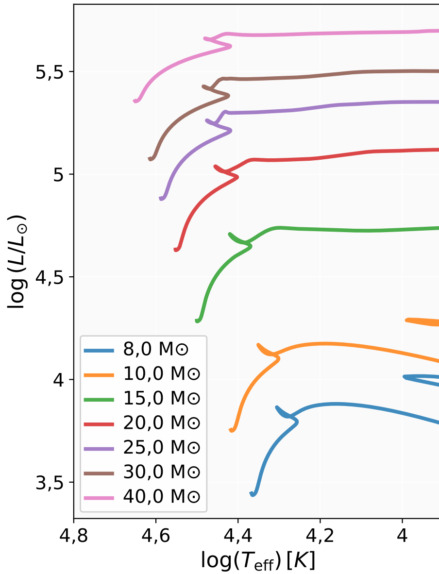
Figura 11.2: Diagrama HR para estrelas de alta massa (8–40 M_{\odot} ).
