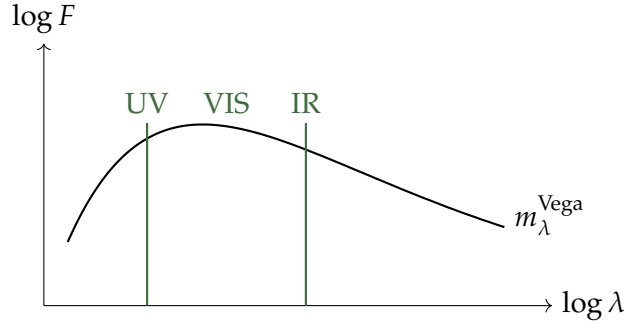
Figura 2.1: Representação esquemática do espectro contínuo de fluxo da estrela Vega (forma ilustrativa, sem escala física), adotado como referência de magnitude zero: m_{\lambda}^{\text{Vega}} = 0 em todo comprimento de onda observado. As faixas ultravioleta (UV), visível (VIS) e infravermelho (IR) estão indicadas.
