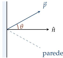
Figura 8.3: Geometria usada na dedução da pressão cinética: uma partícula de momento \vec{p} colide com a parede (normal \hat{n} ) fazendo um ângulo \theta com a normal; a reflexão especular transfere momento \Delta p = 2p \cos \theta para a parede.
