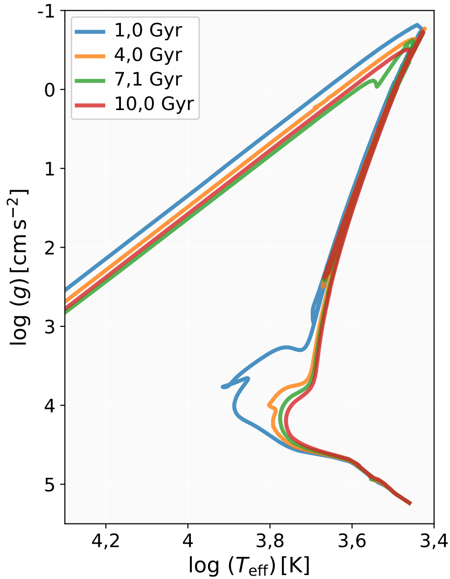
Figura 11.22: Isócronas para metalicidade solar. Observa-se sequência principal mais larga e um ramo de gigantes mais extenso, refletindo maior opacidade.
