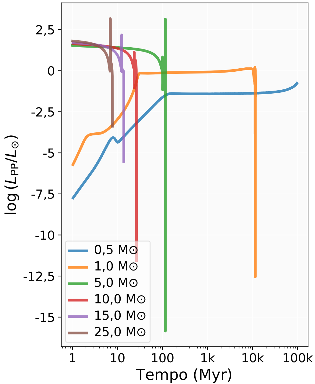
Figura 11.8: Evolução temporal da luminosidade nuclear proveniente da cadeia próton-próton para diferentes massas estelares, evidenciando sua dominância em estrelas de baixa massa e seu rápido declínio em estrelas mais massivas devido à transição para o ciclo CNO.
