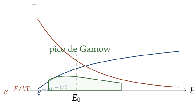
Figura 10.2: O pico de Gamow: a probabilidade de tunelamento ( e^{-bE^{-1/2}} , crescente com E , curva azul) compete com a cauda maxwelliana ( e^{-E/kT} , decrescente, curva vermelha); o produto das duas (região sombreada) forma um pico estreito em E_0 , onde ocorre a maior parte das reações nucleares no interior estelar.
