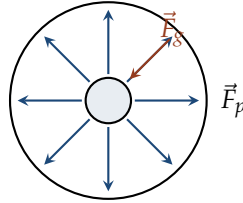
Figura 5.3: Estrela em equilíbrio hidrostático: a força de pressão \vec{F}_p (para fora, em cada direção) equilibra exatamente a força gravitacional \vec{F}_g (para dentro) em cada camada — F_g = F_p .
