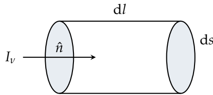
Figura 4.4: Cilindro de fótons de comprimento dl e área de seção ds , usado para deduzir a densidade de energia radiativa.
