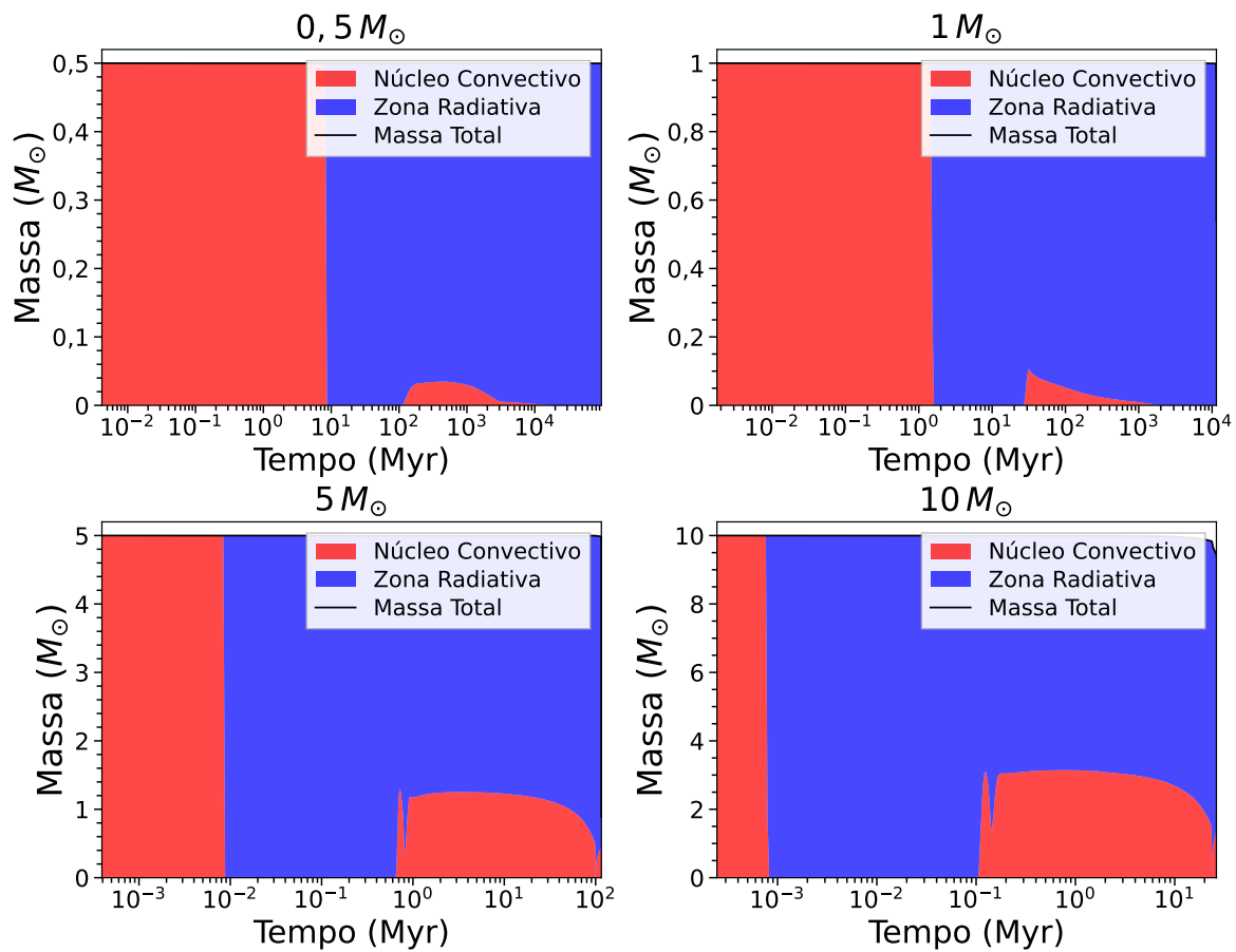
Figura 11.13: Evolução temporal das zonas convectivas (vermelho) e radiativas (azul) para massas entre 0,5 e 10 M_{\odot} . A linha preta representa a massa total, evidenciando perdas por ventos quando presentes.
