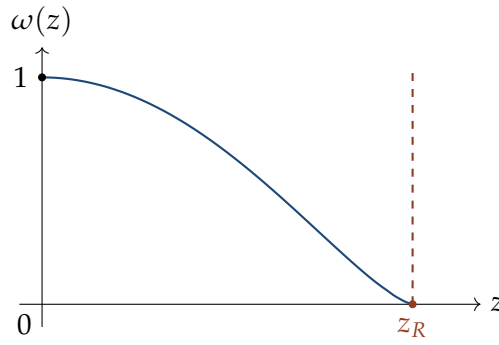
Figura 6.2: Comportamento esquemático da função de Lane–Emden \omega(z) : decresce monotonicamente a partir de \omega(0) = 1 no centro da estrela ( z = 0 ) até se anular no raio politrópico z = z_R (linha tracejada), que marca a superfície estelar.
