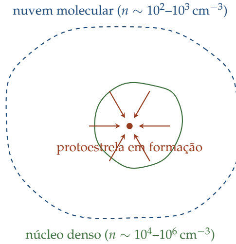
Figura 7.1: Representação esquemática de uma nuvem molecular gigante (contorno tracejado, densidade traçada por CO) contendo um núcleo denso pré-estelar (contorno interno) em colapso gravitacional: à medida que a densidade aumenta localmente, a massa de Jeans [Equação (7.6)] diminui, favorecendo a fragmentação hierárquica discutida no texto.
