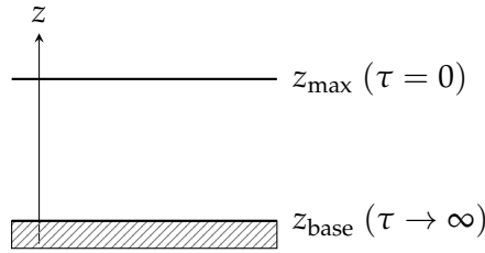
Figura 4.12: Condição de contorno geral em geometria PP: z_{\max} (topo da atmosfera, \tau = 0 ) e z_{\text{base}} (base, tomada como \tau \rightarrow \infty ).
