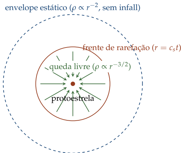
Figura 7.2: Colapso inside-out de Shu (1977): a frente de rarefação, propagando-se a r = c_s t , separa a região interna já em queda livre ( \rho \propto r^{-3/2} , v \propto r^{-1/2} ) do envelope externo ainda estático, com o perfil original da SIS [Equação (7.21)]. A protoestrela cresce a taxa aproximadamente constante [Equação (7.23)] enquanto a frente avança, convertendo progressivamente o núcleo em material em queda.
