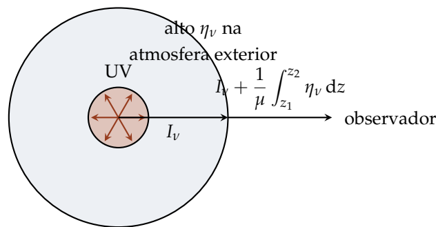
Figura 4.10: Estrutura estrela+nebulosa: a estrela central quente emite radiação UV que ioniza o gás circundante, produzindo alta emissividade \eta_\nu na camada externa (a nebulosa). O feixe I_\nu vindo do disco estelar central atravessa a nebulosa e chega ao observador somado à emissão acumulada ao longo do caminho, conforme a Equação (4.68).
