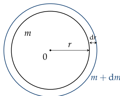
Figura 5.1: Casca esférica de espessura dr a uma distância r do centro da estrela: a massa contida até r é m , e a massa contida até r + dr é m + dm .
