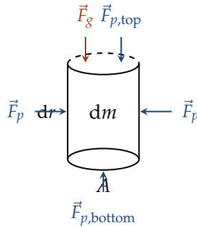
Figura 5.4: Elemento cilíndrico de gás usado para deduzir o equilíbrio hidrostático: força gravitacional \vec{F}_g e forças de pressão no topo, na base e nas laterais — estas últimas se cancelam pelo Teorema de Stevin.
