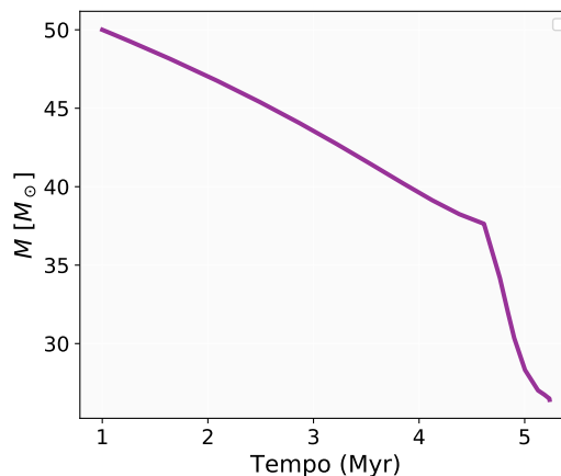
Figura 11.28: Perda de massa contínua e intensa, atingindo 47% da massa inicial.
