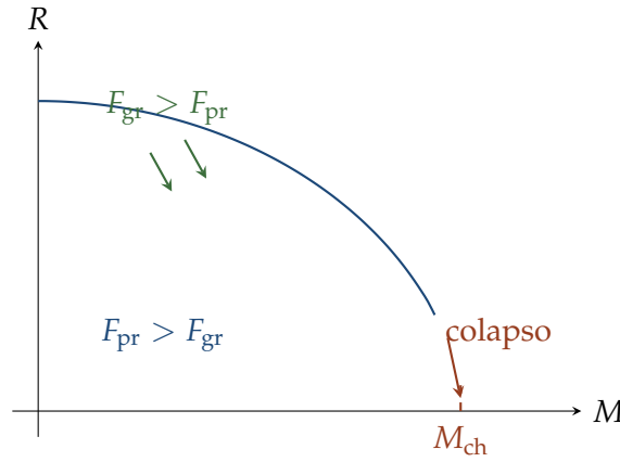
Figura 9.2: Relação massa-raio esquemática de anãs brancas: curva decrescente separando a região estável ( F_{\text{pr}} > F_{\text{gr}} , sustentada por degenerescência eletrônica) da região instável ( F_{\text{gr}} > F_{\text{pr}} ), com o colapso ocorrendo ao se aproximar da massa de Chandrasekhar, M_{\text{ch}} , no eixo horizontal.
