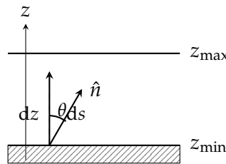
Figura 4.8: Deslocamento ds ao longo da direção \hat{n} , com componente vertical dz = ds \cos \theta .
