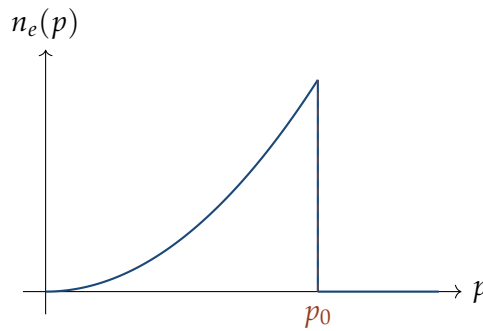
Figura 8.2: Densidade de elétrons por intervalo de momento, n_e(p) , para um gás totalmente degenerado em T = 0 : cresce \propto p^2 até p_0 e cai abruptamente a zero acima desse valor — todos os estados até p_0 estão ocupados, e nenhum além dele.
