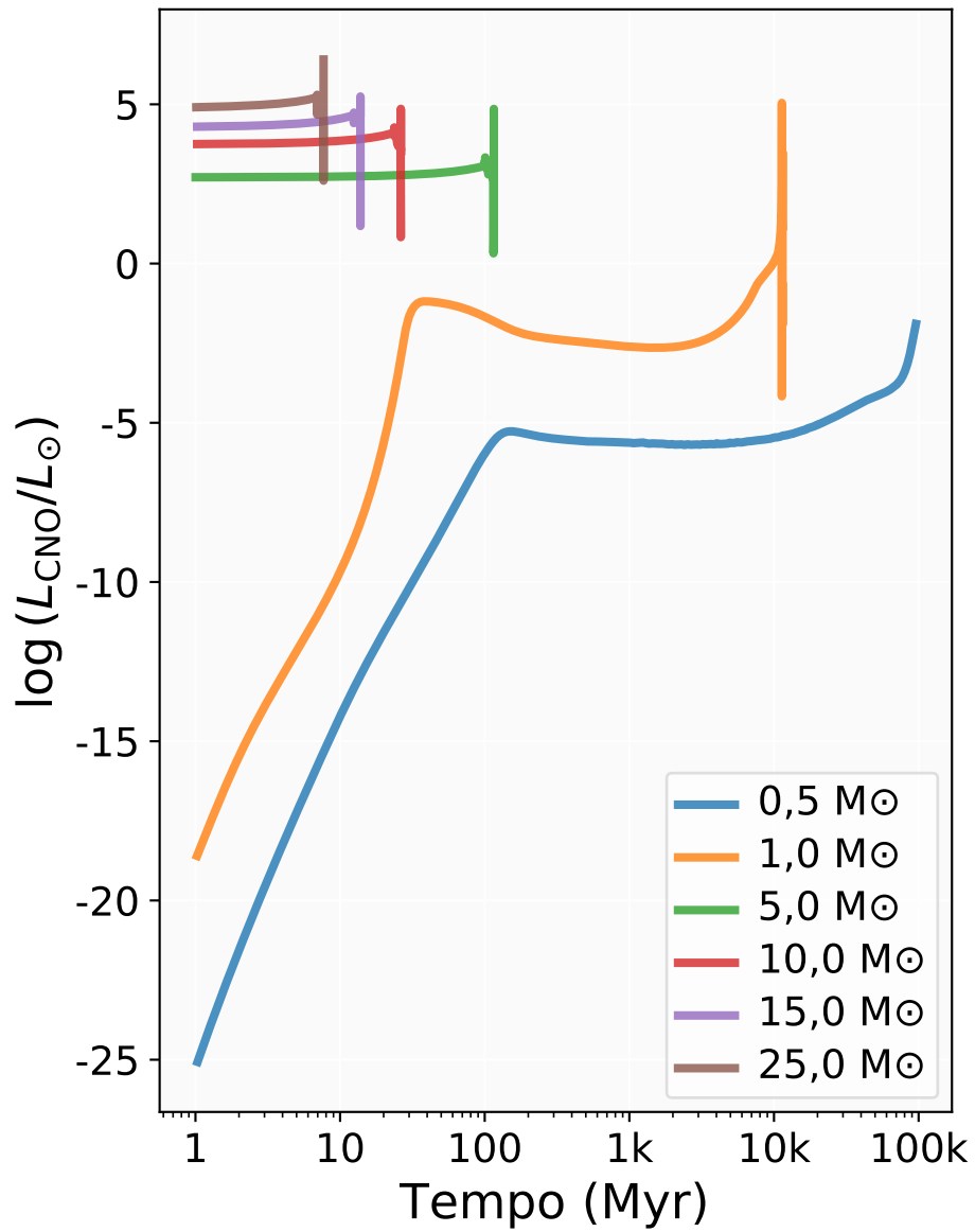
Figura 11.9: Contribuição temporal do ciclo CNO para a geração de energia nuclear em estrelas entre 0,5 e 25 M_{\odot} , destacando sua sensibilidade extrema à temperatura e seu papel dominante na sequência principal de estrelas intermediárias e massivas.
