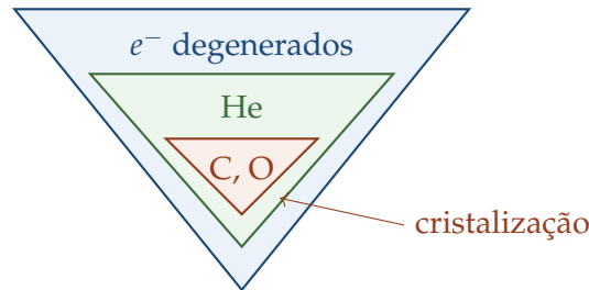
Figura 9.1: Corte transversal esquemático da estrutura em camadas de uma anã branca: camada externa de elétrons degenerados, camada de hélio, e núcleo de carbono e oxigênio, onde ocorre a cristalização discutida no Capítulo 8.
