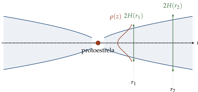
Figura 7.6: Estrutura vertical de um disco (fora de escala): H(r) cresce com o raio (disco flaring , Seção 7.8), e em cada raio a densidade segue o perfil gaussiano \rho(z) \propto \exp(-z^2/2H^2) [Equação (7.39)], ilustrado à esquerda em r_1 .
