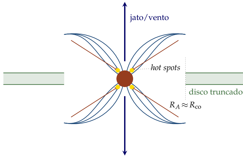
Figura 7.8: Acréscimo magnetosférico (fora de escala): o disco viscoso (Seção 7.8) é truncado em R_A [Equação (7.54)], próximo a R_{co} [Equação (7.55)]; dentro dele, o gás é canalizado em colunas de acréscimo até hot spots (Seção 7.9), enquanto ventos/jatos são lançados ao longo do eixo (Seção 7.9).
