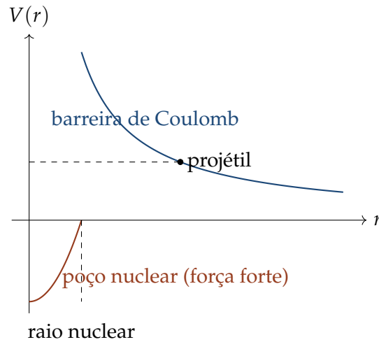
Figura 10.1: Barreira de Coulomb: energia potencial em função da distância r entre os núcleos. Dentro do raio nuclear, a força forte domina, formando um poço atrativo; fora dele, domina a repulsão coulombiana entre as cargas positivas, formando a barreira. A energia cinética típica do projétil (linha tracejada) fica bem abaixo do topo da barreira, exigindo tunelamento quântico para que a reação ocorra.
