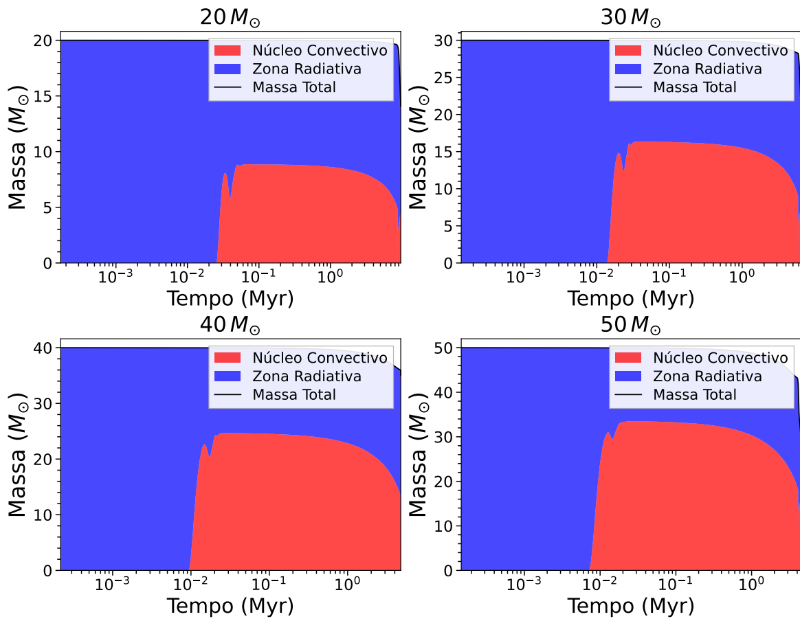
Figura 11.14: Zonas convectivas para estrelas massivas ( 20\text{--}50 M_{\odot} ). Nota-se o núcleo convectivo crescente e a perda de massa (linha preta) que modifica a estrutura interna.
