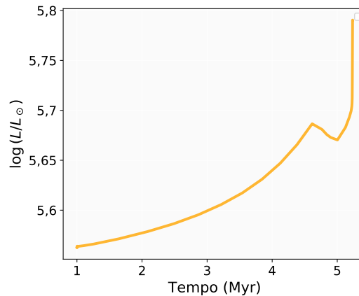
Figura 11.25: Evolução da luminosidade ao longo da simulação. A luminosidade aumenta de forma quase monótona, característica do aumento contínuo da taxa de queima nuclear.
