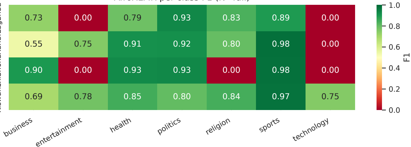
AfroXLMR per-class F1 (N=full)
