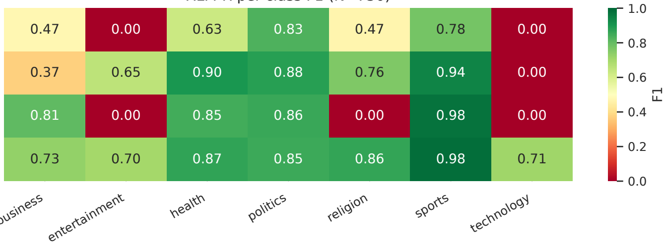
XLM-R per-class F1 (N=750)
