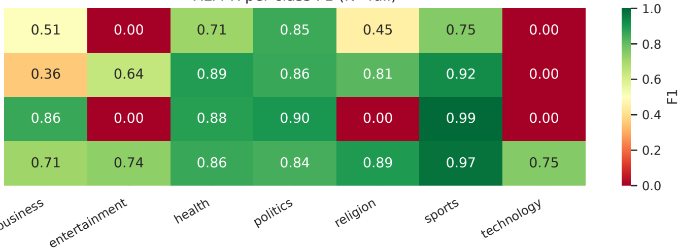
XLM-R per-class F1 (N=full)
