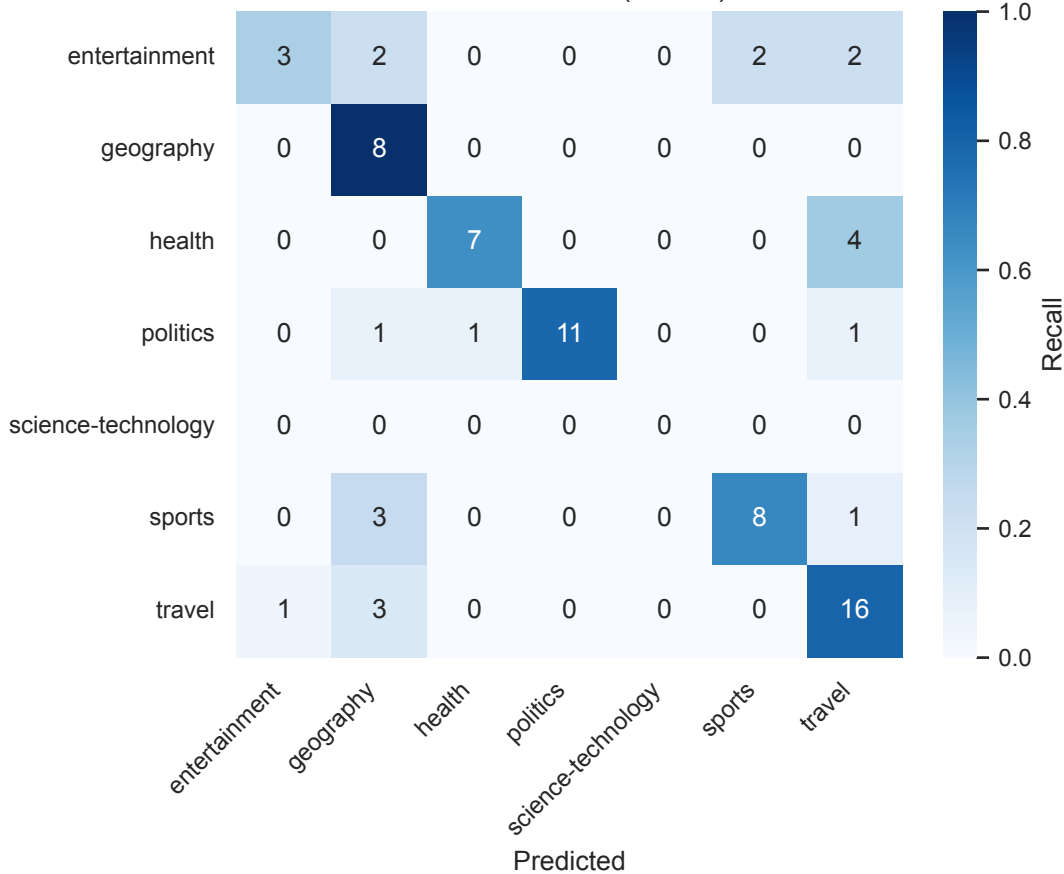
XLM-R - Hausa (N=500)
