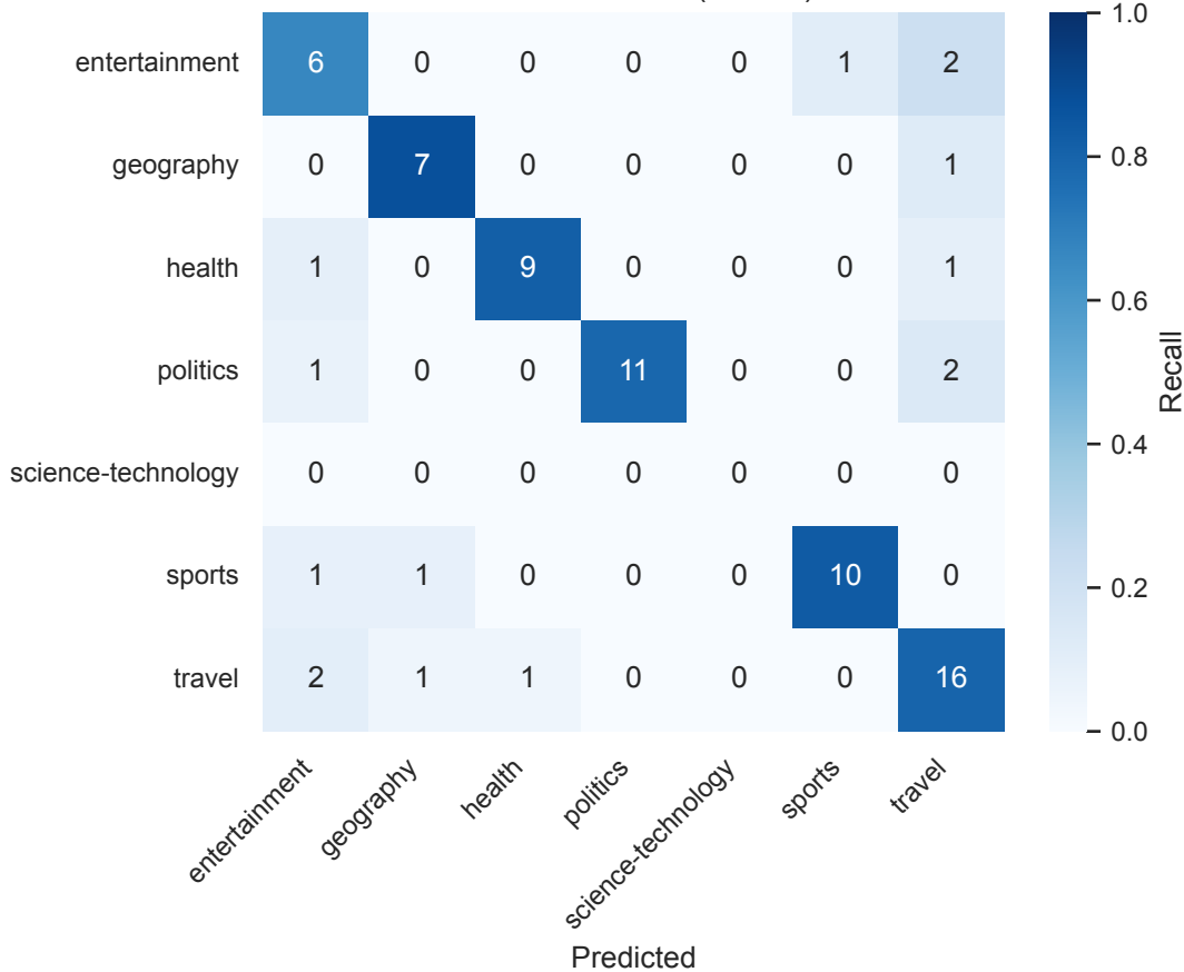
XLM-R - Swahili (N=500)
