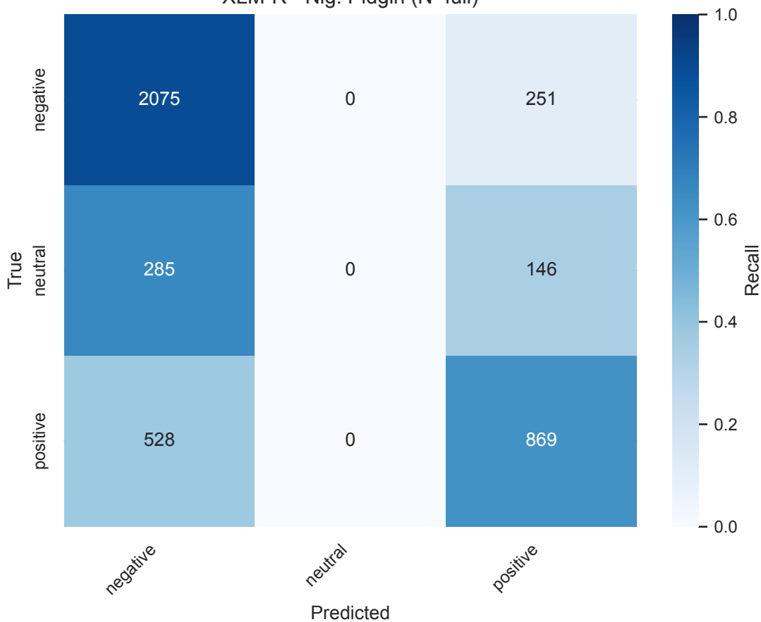
XLM-R - Nig. Pidgin (N=full)
