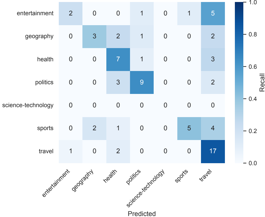
AfroXLMR - Luganda (N=full)
