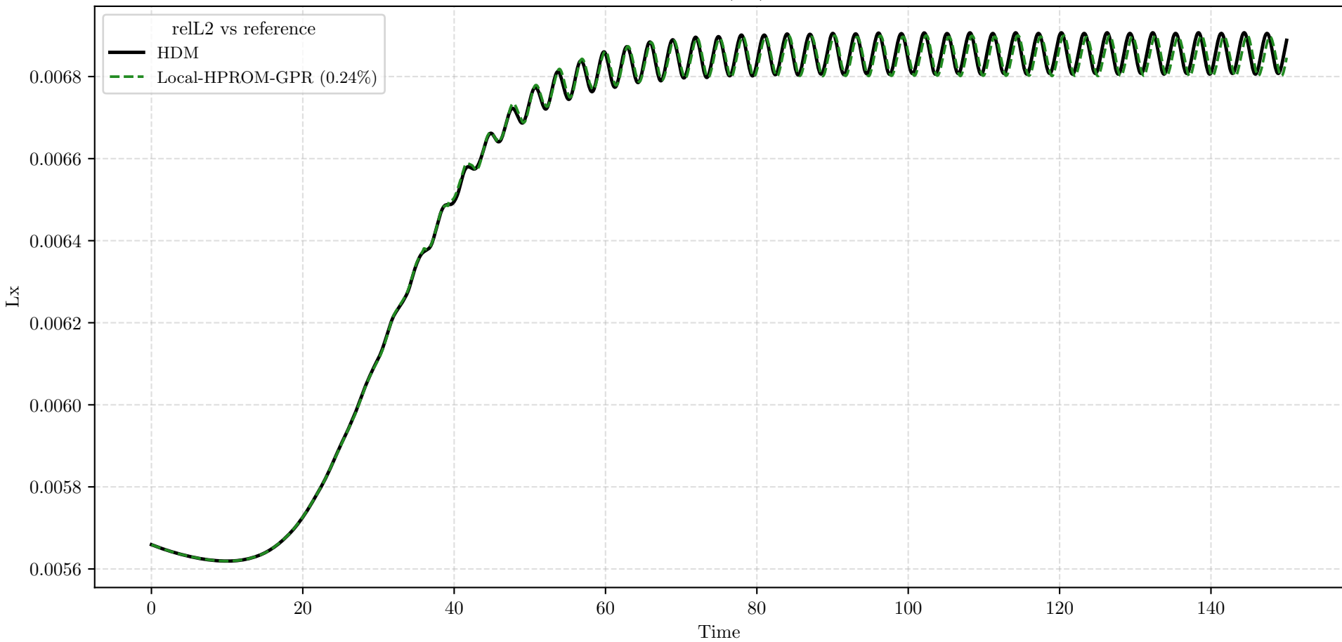
Drag ( Lx )
