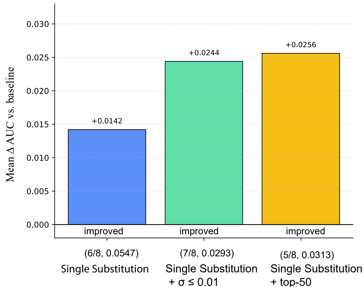
A. BigTB Benchmark
