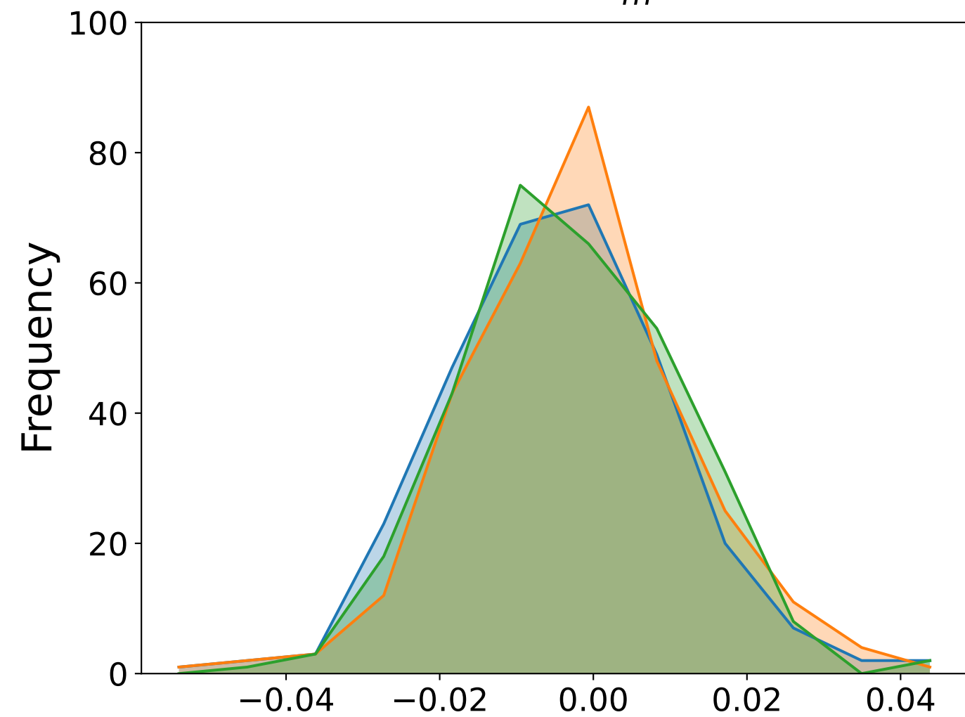
(d) C_c(x_c^*)
