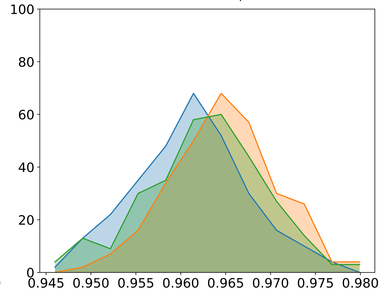
(f) CEC_{0,l',z}
