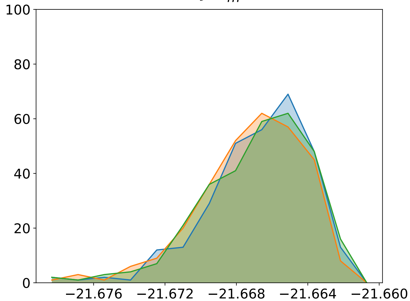
(e) J(x_c^*)
