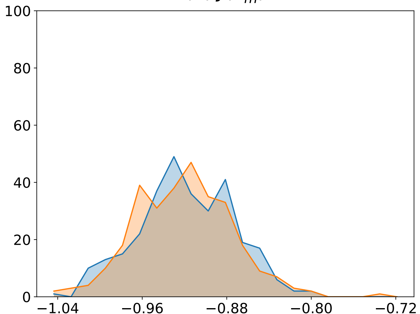
(e) J(x_c^*)
