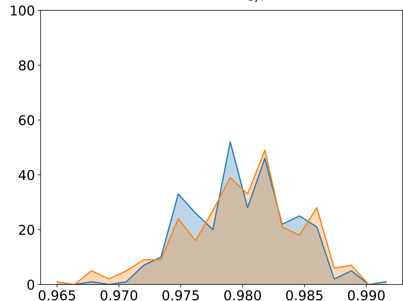
(f) CEC_{0,l',z}
