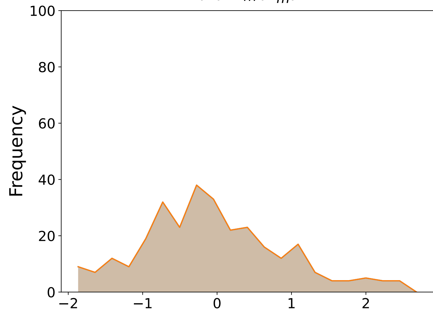
(d) C_c(x_c^*)
