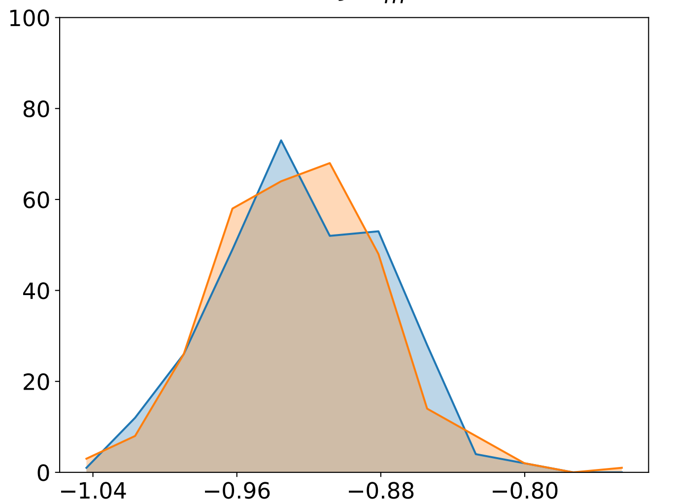
(e) J(x_c^*)
