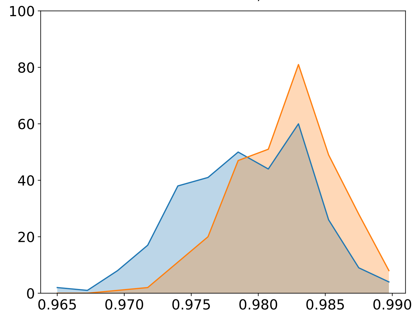
(f) CEC_{0,l',z}
